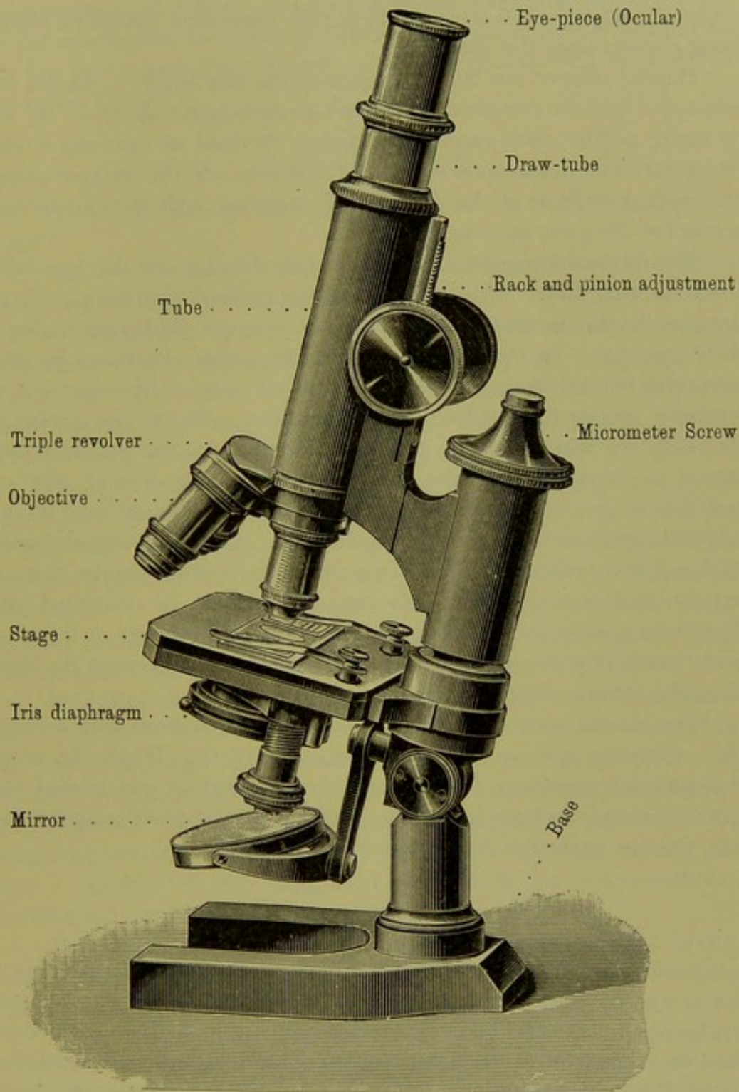
FIG. 1.—LEITZ MICROSCOPE. STAND II ( \frac{1}{2} actual size).
