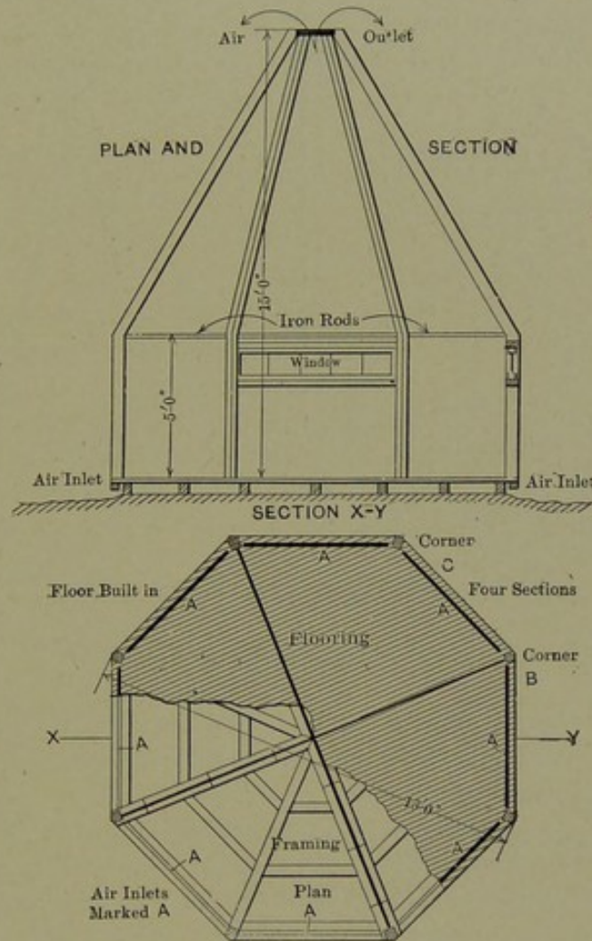
FIG. 118.—The Gardiner tent.
