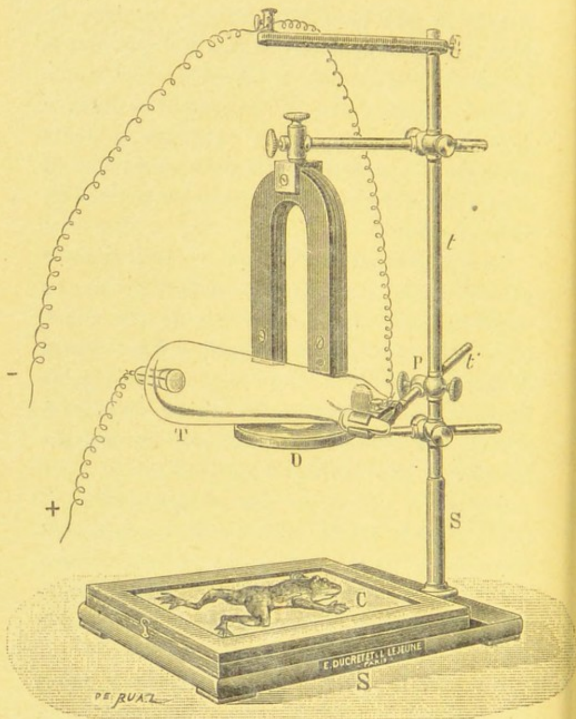
FIG. 22. — Appareil à diaphragme construit par M. Ducretet, pour l'obtention des épreuves par les rayons X. T , ampoule de Crookes surmontée d'un aimant; D , diaphragme; C , châssis renfermant la plaque photographique.
