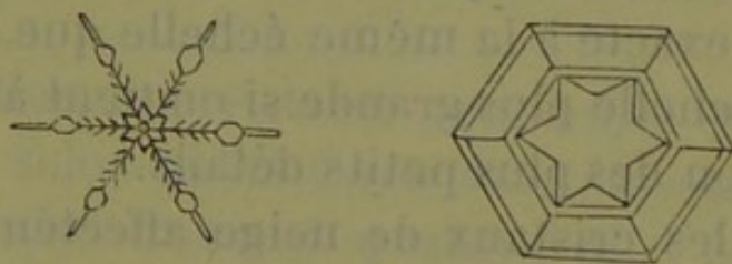
Fig. 11. — Forme des cristaux de neige.
