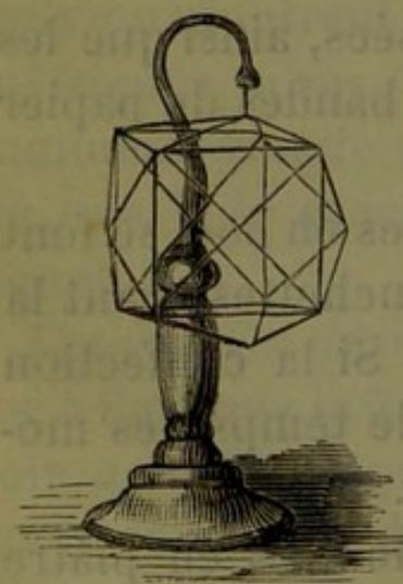
Fig. 9. — Modèle de cristal en fil de fer.
