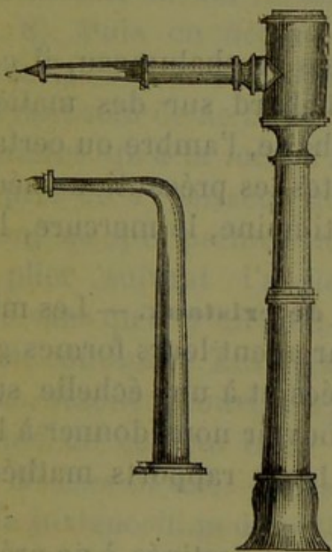
Fig. 6. — Chalumeaux.
