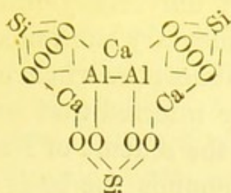
Garnet (Lime Alumina).
