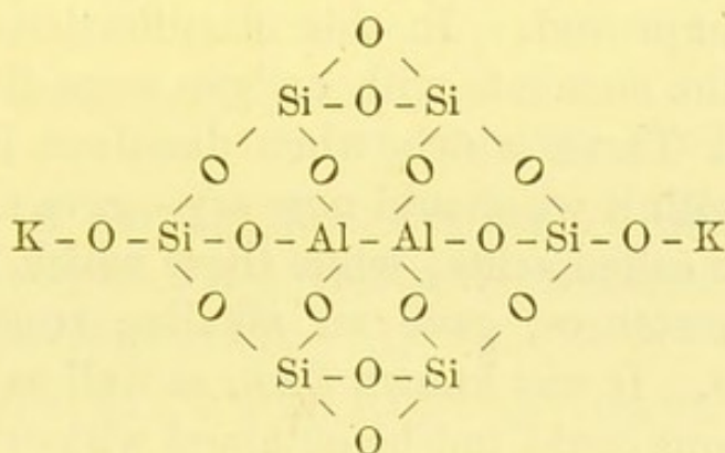
Feldspar (Orthoclase).
