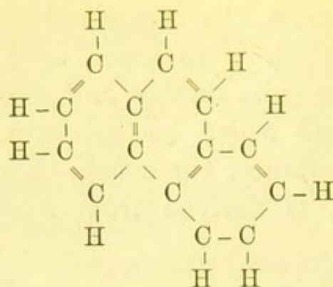
Anthracene.
