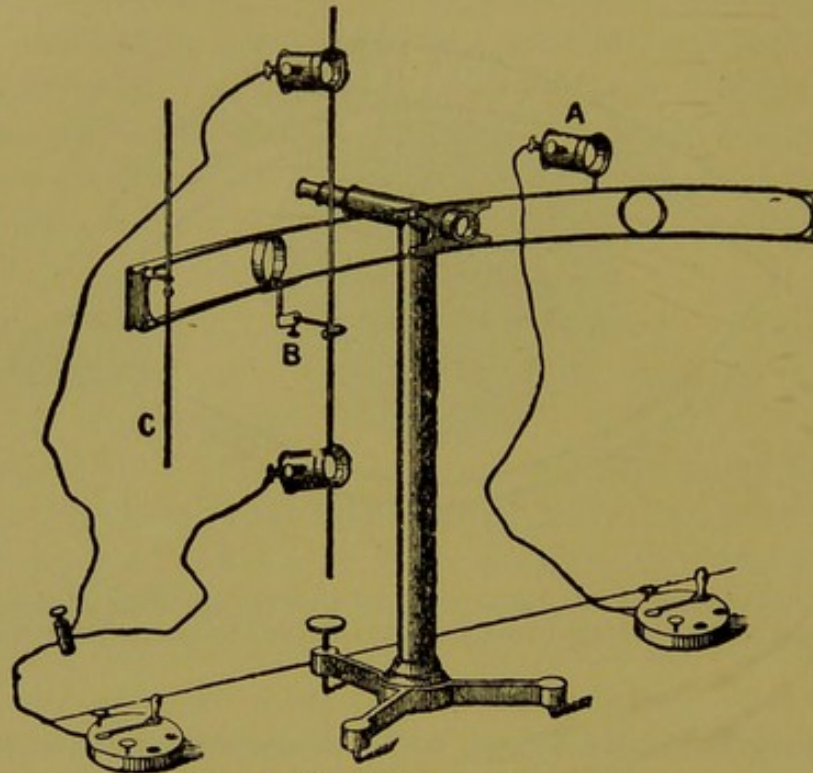
Fig. 32—The Ophthalmophakometer.
