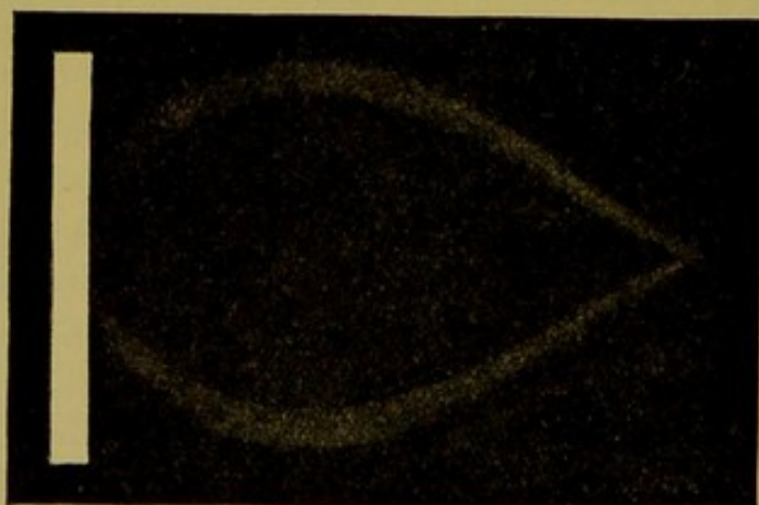
Fig. 106a. — Entoptic phenomenon.
