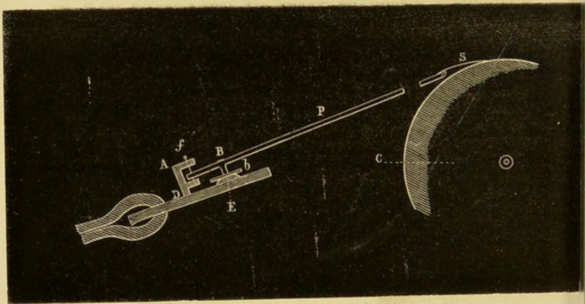
Fig. 98. — Appareil pour enregistrer le mouvement des cils vibratiles. — E, lame de liège portée sur un support à mâchoires. — AE, armature verticale. — f , axe du mouvement formé par une épingle. — P, Tige de paille portant un style en S. — B, tige de paille à angle droit avec la paille porte-style. — b , lamette de verre en contact avec la membrane ciliée. — C, cylindre enregistreur.
