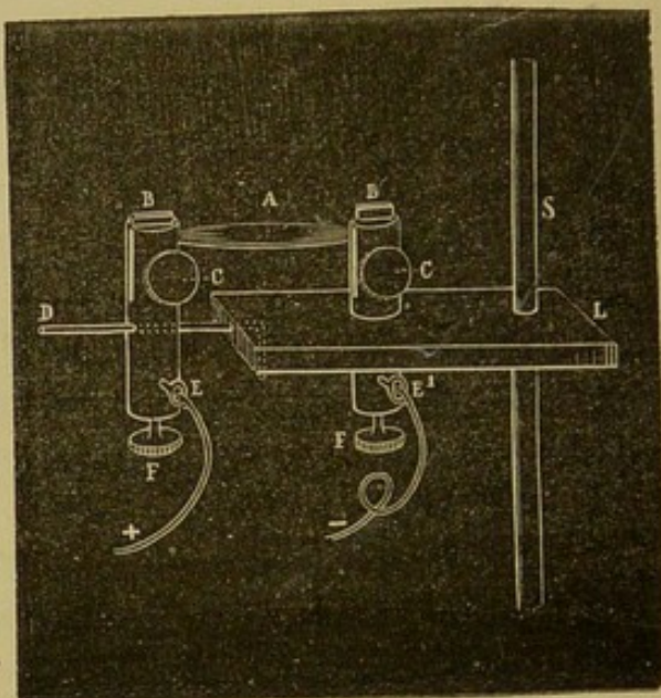
Fig. 20. — Appareil pour l'excitation d'un muscle. S, support. L, lame de liège enduite de cire d'Espagne portant la borne B', qui reçoit le fil négatif E'. — D, tige de fer portant la seconde borne B, qui reçoit le fil positif, E. A, Muscle couturier de la grenouille tendu entre les deux bornes. F F, vis de pression destinées à fixer les fils E E'; — C C, vis de pression destinées à maintenir les chefs du muscle entre les mors des deux bornes.
