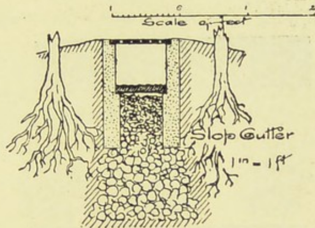
FIG. 26.—FILTRATION GUTTER.
