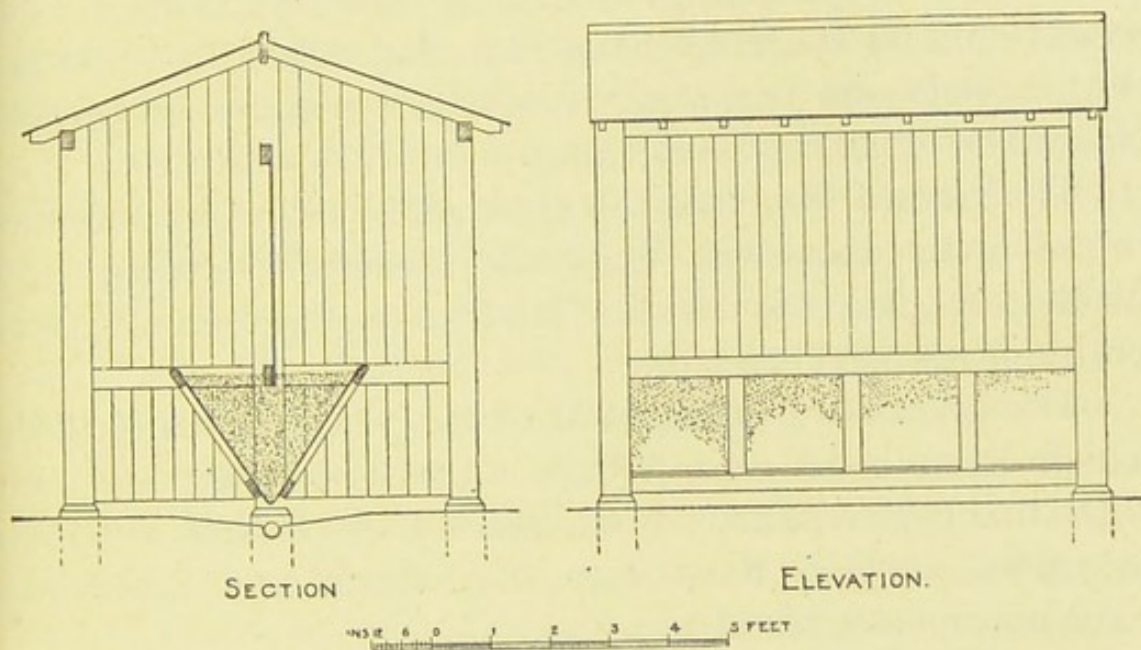
FIG. 21.—DRY URINAL.
