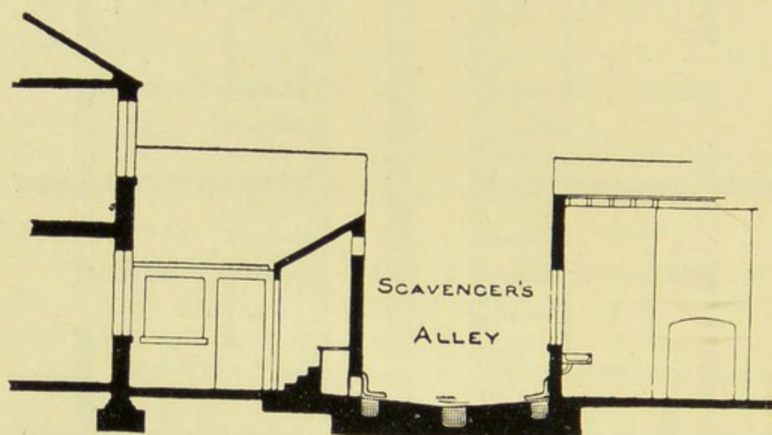
FIG. 30.—SECTION A-A.
