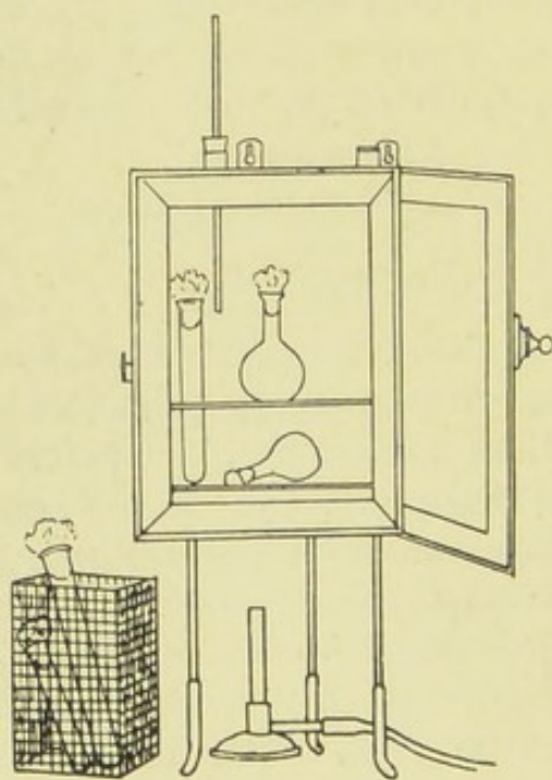
FIG. 2.—Hot-air steriliser.
