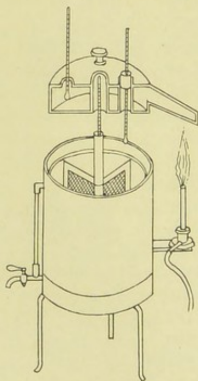
FIG. 5.—Steriliser for blood serum.
