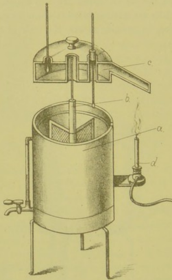
FIG. 53.—Slow steriliser for blood serum.
