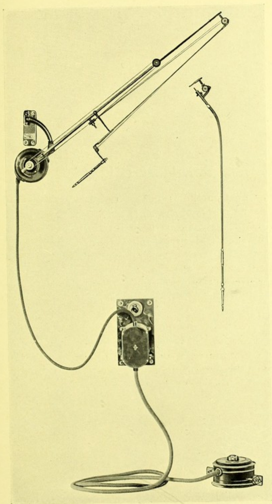
The S. S. White Swivel-Bracket Dental Engine
