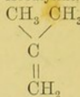
Isobutylene.
