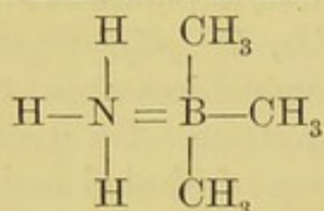
Ammonio-boron Methide.
