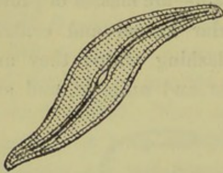
NAVICULA HIPPOCAMPUS.
