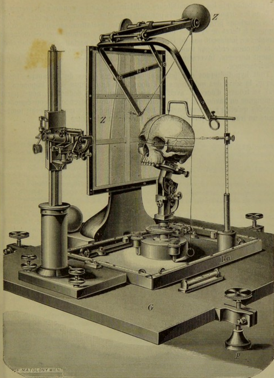
Fig. 25. — CATHÉTOMETRE CRANIMÉTRIQUE OPTIQUE monté, du professeur Benedikt (dessin d'après une photographie).
