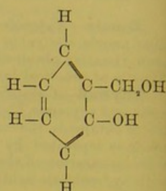
Saligenin (alphenol).
