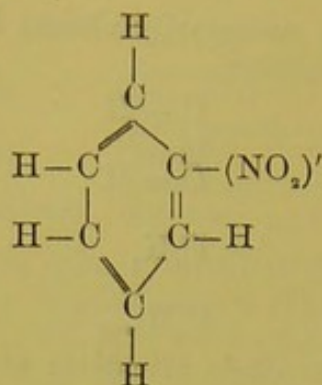
Nitro-benzene.
