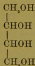
Erythrite.
