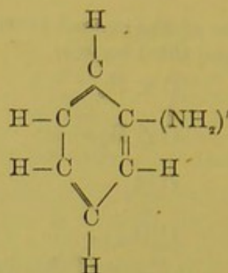
Amido-benzene (aniline).
