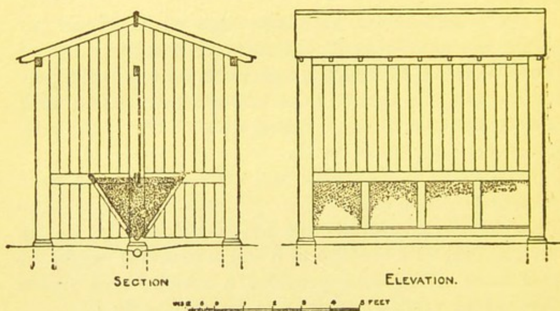
FIG. 9.—DRY URINAL.
