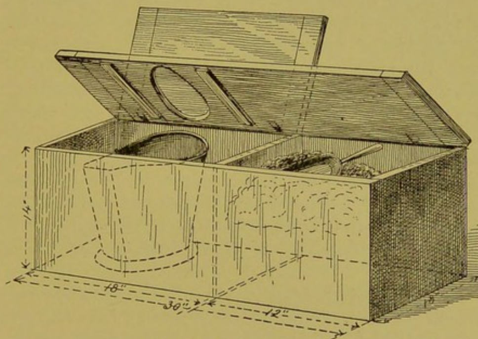
FIG. 42.—Dry-earth closet.
