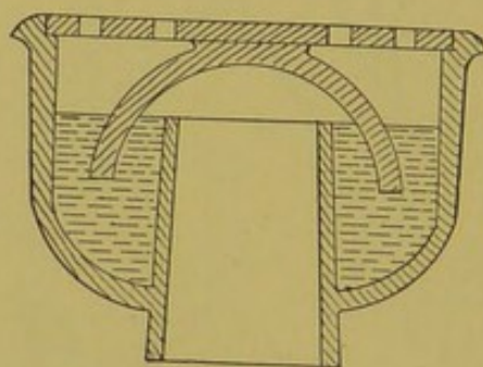
FIG. 37.—Bell-trap.
