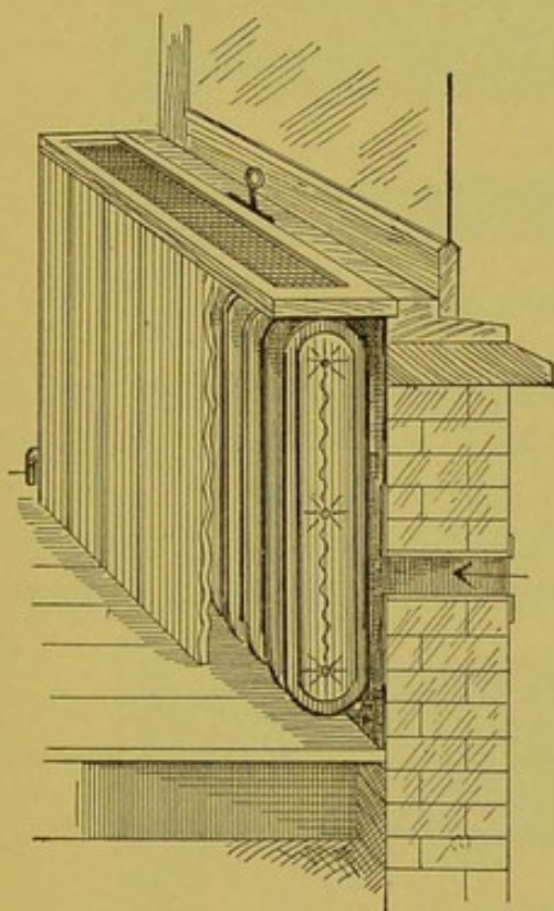
FIG. 9.—Wall air inlet.
