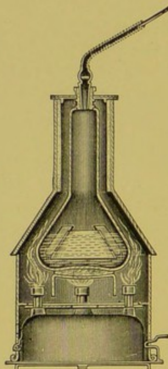
FIG. 62.—Formaldehyd gas regenerator.
