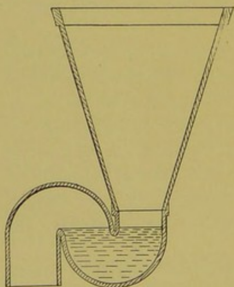
FIG. 31.—Hopper closet.
