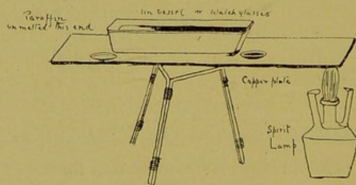
Fig. 8. Simple Embedding Apparatus
