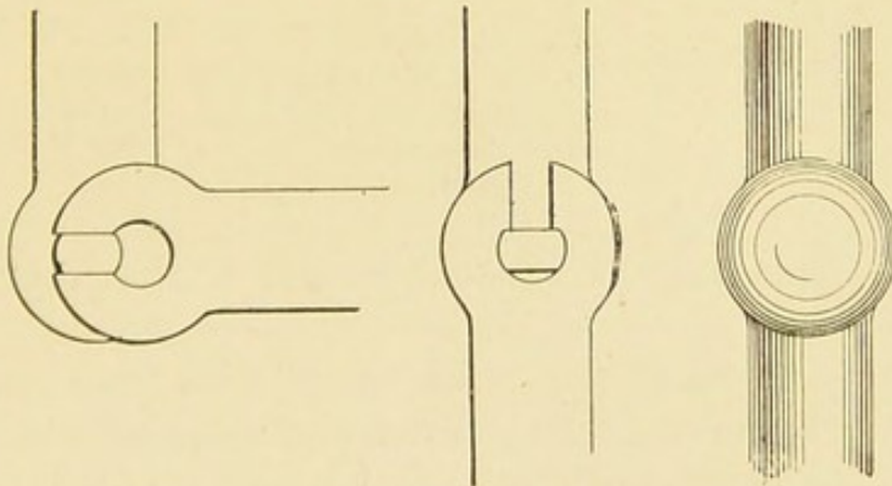
Fig. 39.—Detachable Joint.
