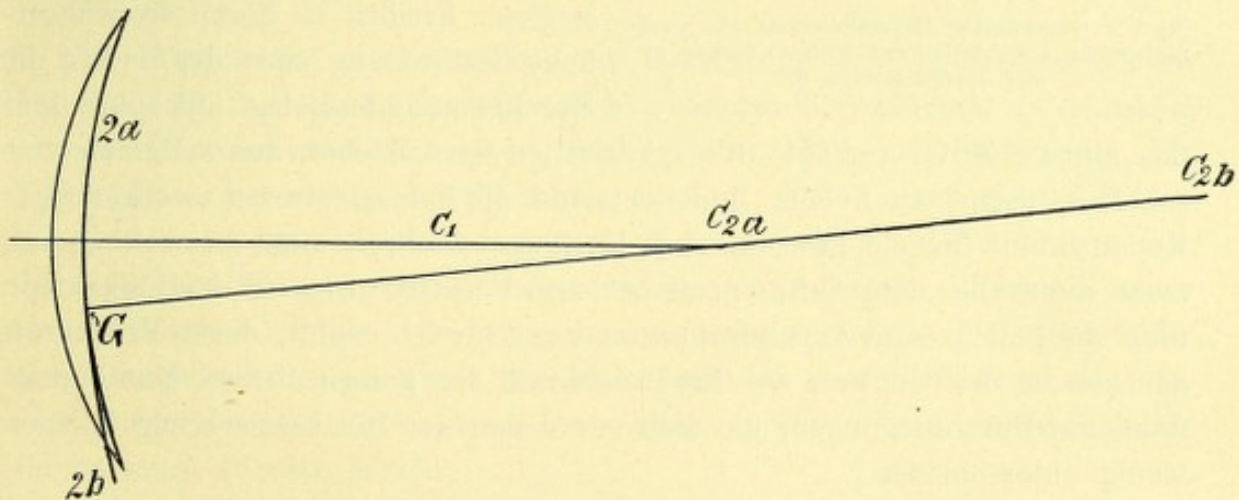
Doppelfokusglas mit sprunglosem Übergang außerhalb der Achse bei G .
