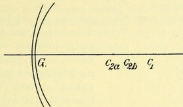
Doppelfokusglas mit sprunglosem Übergang in der Achse bei G .
