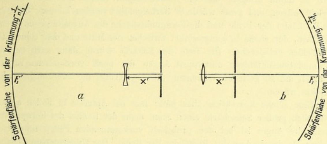
Schematische Darstellung der Lage von Schärfen- oder Bildfläche und Blende mit dem Abstand x' für eine zerstreuernde sammelnde Korrektionsbrille mit deutlichem Blickfelde.
