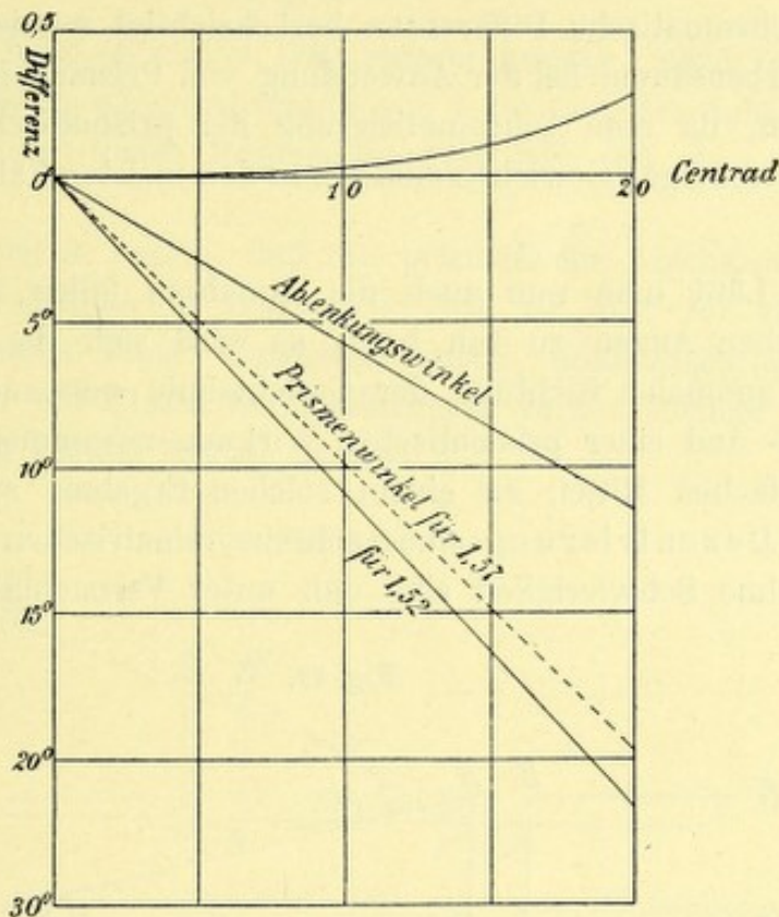
Graphische Darstellung der Prismenwinkel \alpha , des Ablenkungswinkels \epsilon in Graden, der Differenz (Maßzahl prdptr - Maßzahl ctrd) in Dezimalen für 0 bis 20 ctrd.
