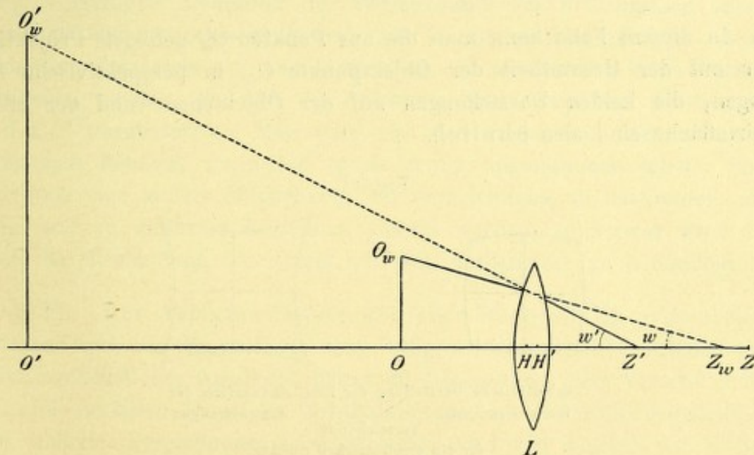
Schematische Darstellung des Strahlenganges für die Definition der Verzeichnung eines Brillenglases bei endlichen Neigungswinkeln w , w' des Hauptstrahls.
