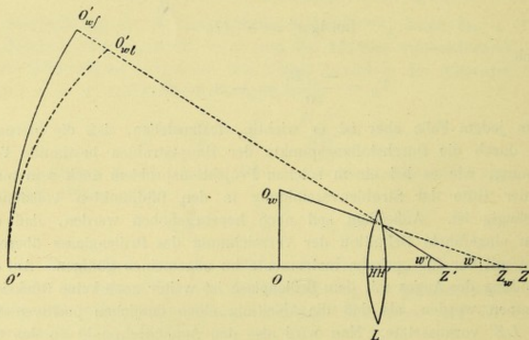
Schematische Darstellung des Strahlenganges für den Astigmatismus längs einem unter w, w' geneigten Hauptstrahl endlicher Neigung.
