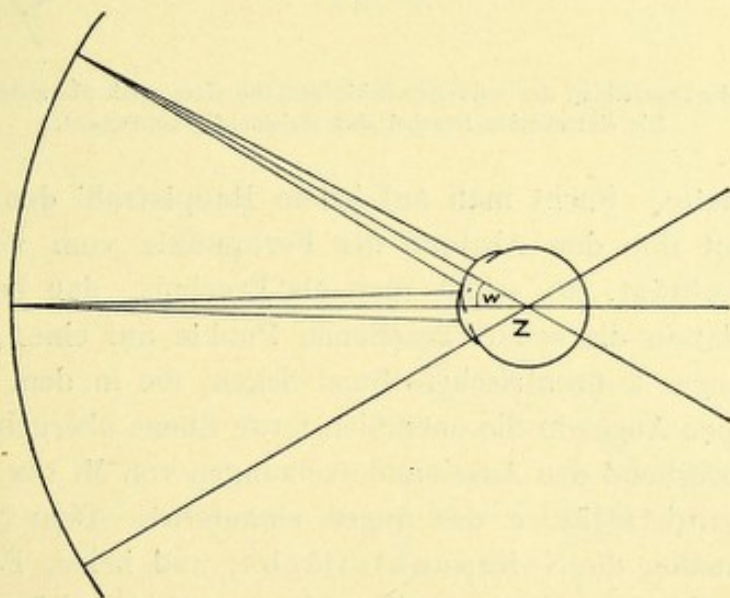
Schematische Darstellung der reellen Schärfenfläche eines stark kurzsichtigen Auges. Die eintretenden Büschel sind gleichmäßig divergent.
