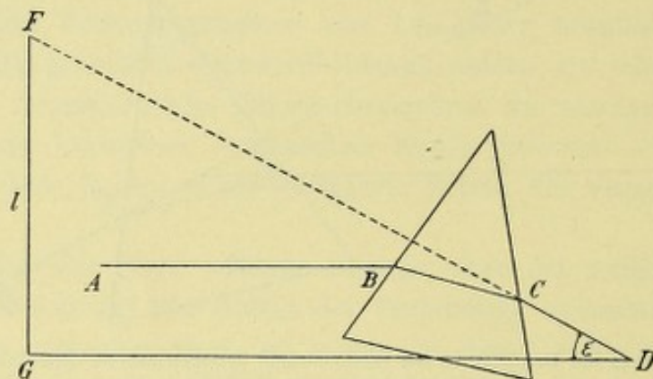
Schematische Darstellung des PRENTICESchen Meßverfahrens.
