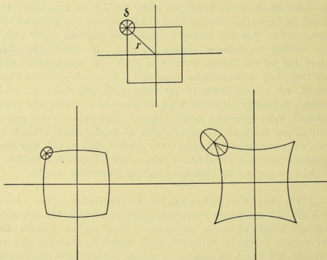
Schematische Darstellung der Erscheinungsform eines exzentrisch angenommenen Kreises bei tonnenförmiger Verzeichnung kissenförmiger
