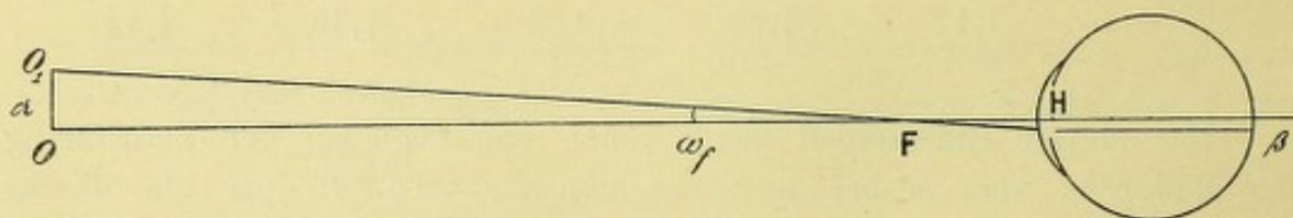
Der Fokalkpunktswinkel \omega_f zur Bestimmung der absoluten Sehschärfe S .
