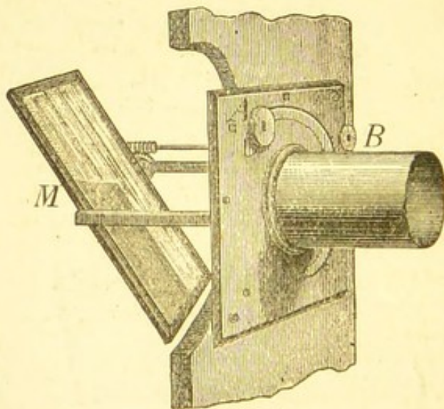
A Heliostat.
