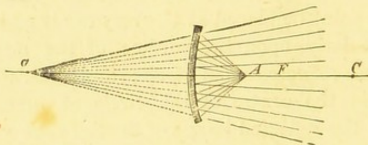
Conjugate foci.
