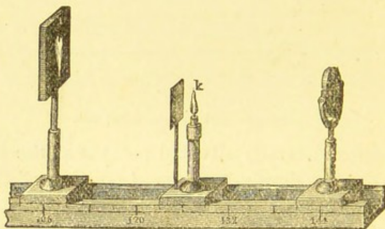
Real image.
