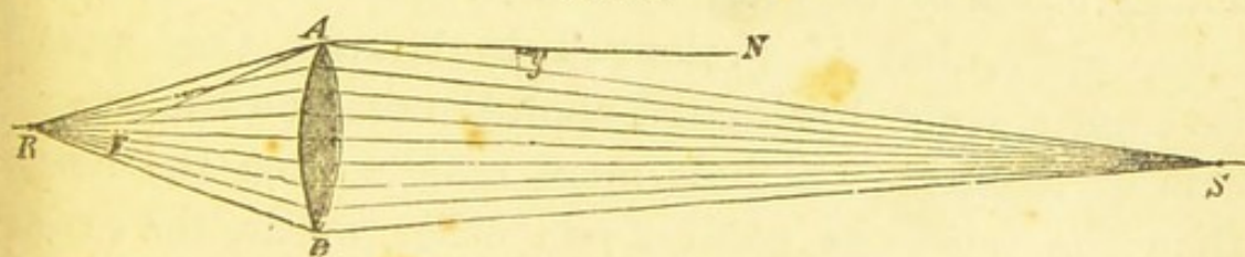
Conjugate foci.
