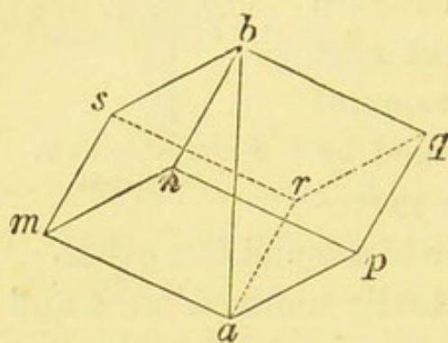
Rhombohedron.
