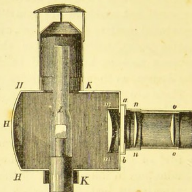
Magic Lantern.
