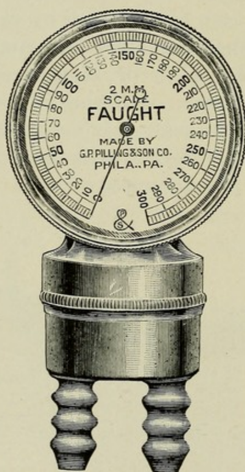
FIG. 9.—Pocket Indicator. Actual size.
