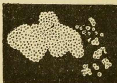
Fig. 9. Mikrokokkenkolonien 1000|1 (ÖRTEL).
