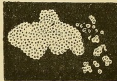
Fig. 9. Mikrokokkenkolonien 1000|1 (ÖRTEL).
