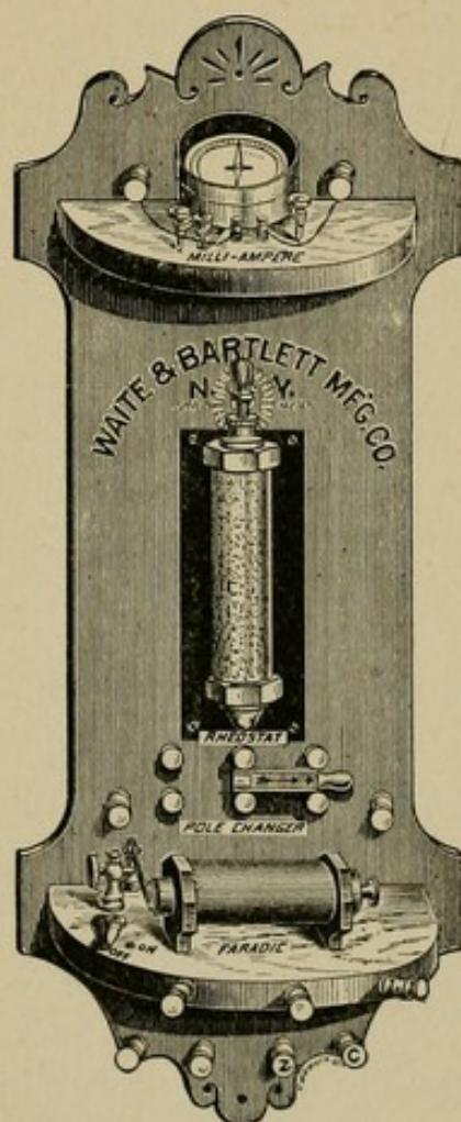
FIG. 19.—Milliampèremeter and Rheostat.
