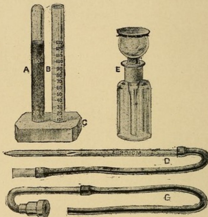
FIG. 9.—HALDANE'S HÆMOGLOBINOMETER.
