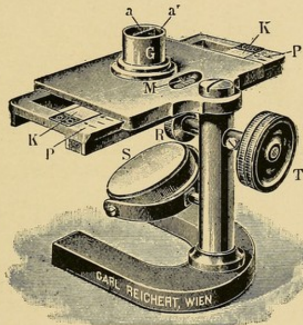
FIG. 10.—VON FLEISCHL'S HÆMOGLOBINOMETER.
