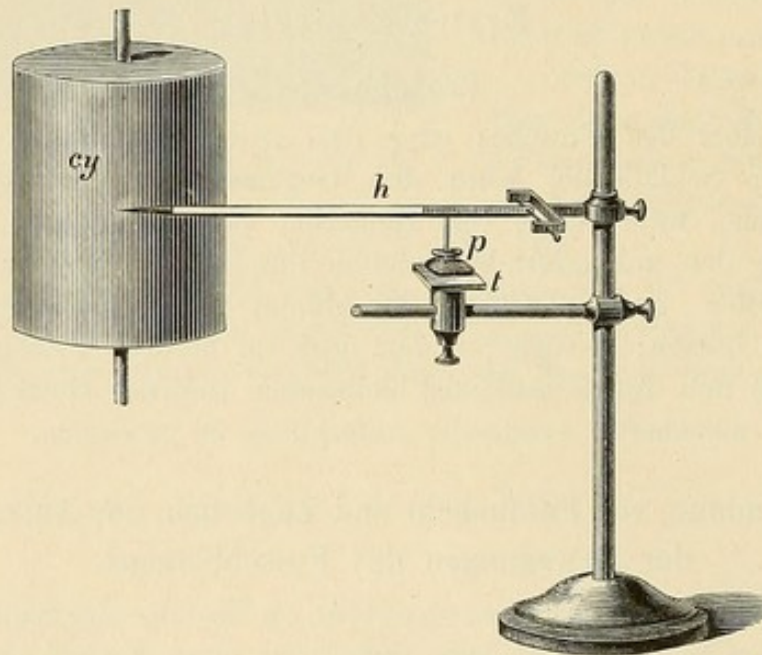
Fig. 136. Fühlhebel für das Froschherz ( \frac{1}{3} nat. Gr.).
