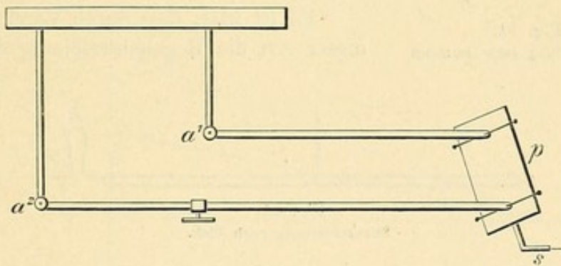
Fig. 33. Geradföhrung der Schreibspitze (Vierordt.)
