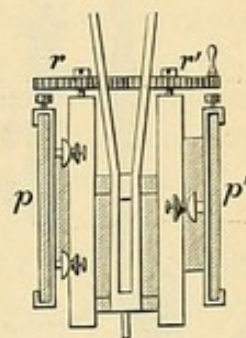
Fig. 232. Das Plattenpaar des Pendelmyographions. ( \frac{1}{2} nat. Gr.)
