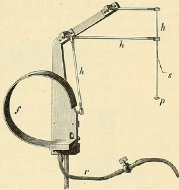
Fig. 173. Flachfedermanometer (Federkymographion) von Fick. ( \frac{1}{4} nat. Gr.)
