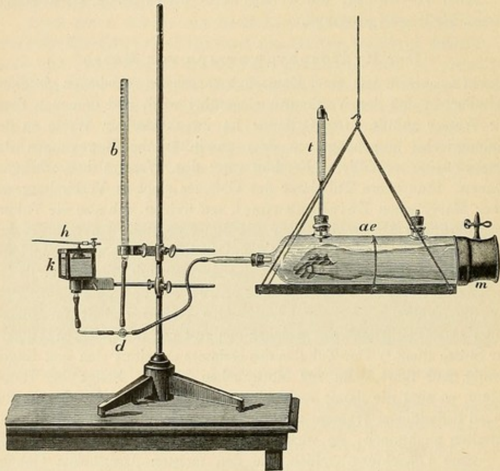
Fig. 199. Plethysmograph nach Kronecker. ( \frac{1}{8} nat. Gr.)
