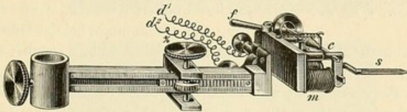
Fig. 123. Signal Deprez nach Verdin. ( \frac{2}{3} nat. Gr.)
