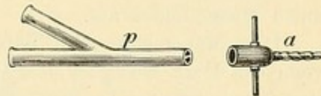
Fig. 144. Perfusionscanüle von Williams. (nat. Gr.)
