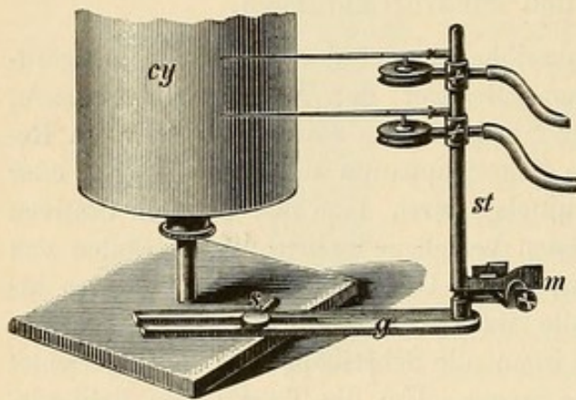
Fig. 54. Anbringung von Schreibapparaten am Cylinder.
