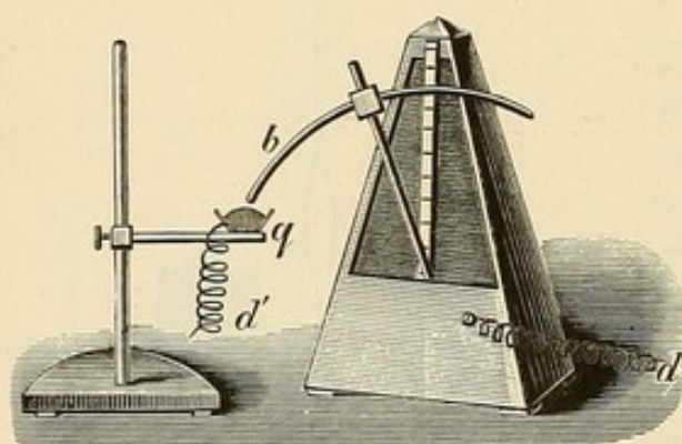
Fig. 95. Stromunterbrechendes Metronom.
