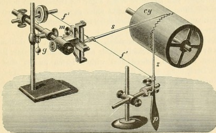
Fig. 223. Zwerchfellhebel von Kronecker und Marckwald.
