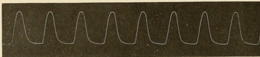
Fig. 137. Pulse des ausgeschnittenen Froschherzens, vermittelt des Fühlhebels aufgezeichnet.
