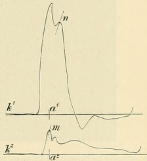
Fig. 89. Intrakardialer Druck ( k^1 ) und arterieller Blutdruck ( k^2 ).
