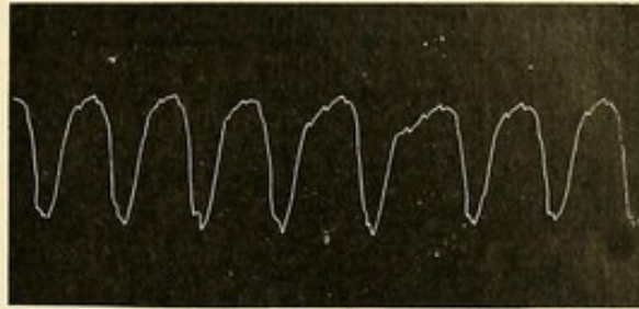
Fig. 217. Kaninchen. Athmung vermittelt der Oesophagussonde aufgeschrieben.
