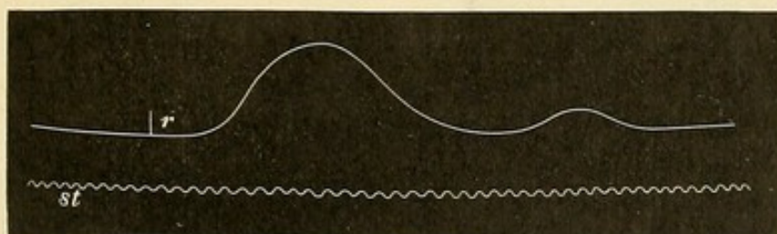
Fig. 233. Zuckungcurve eines Muskels, auf die Platte des Pendelmyographions gezeichnet.
