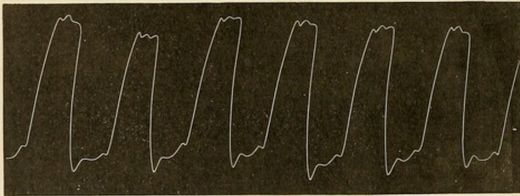
Fig. 158. Spitzenstosscurve vom Menschen.
