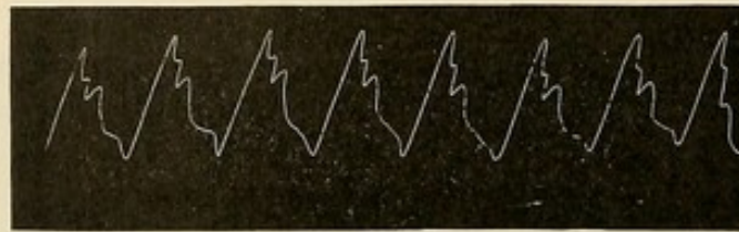
Fig. 193. Karotidenpuls (Kardiograph).
