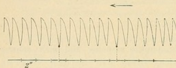
Fig. 76. Athemungscurven mit Chronogramm.
