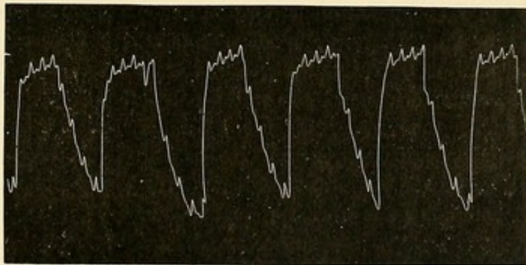
Fig. 218. Kaninchen. Mediastinale Druckschwankungen. Knoll'sche Canüle.
