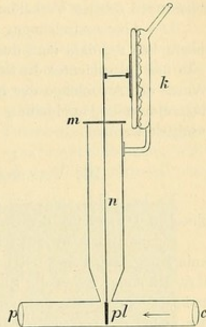
Fig. 203. Haemodromograph mit Luftübertragung.
