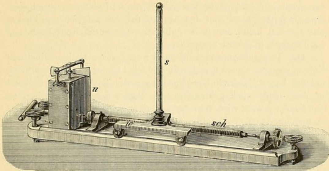
Fig. 18. Marey's Chariot automoteur (nach Verdin).
