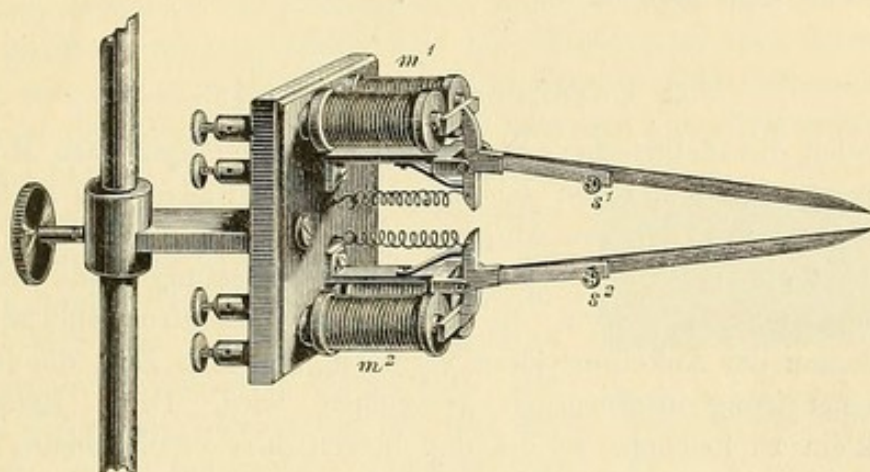
Fig. 125. Elektrisches Doppelsignal (fast nat. Gr.).
