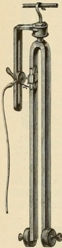
Fig. 106. Stimmgabel mit Auf- nahmekapsel von Marey.
