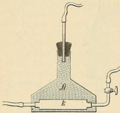
Fig. 174. Metallmanometer von Marey.
