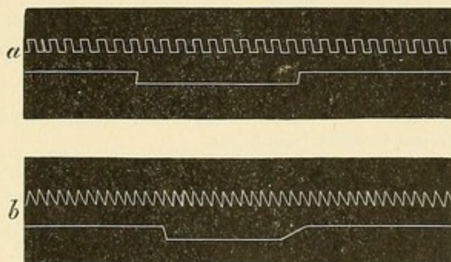
Fig. 126. Zeitmarken und Signale des Doppel-Markirmagnets. In a und b sind die unteren Linien Signalcurven; die chronographischen Aufzeichnungen über denselben entsprechen bei a Doppelsekunden, bei b \frac{1}{50} Sekunden.
