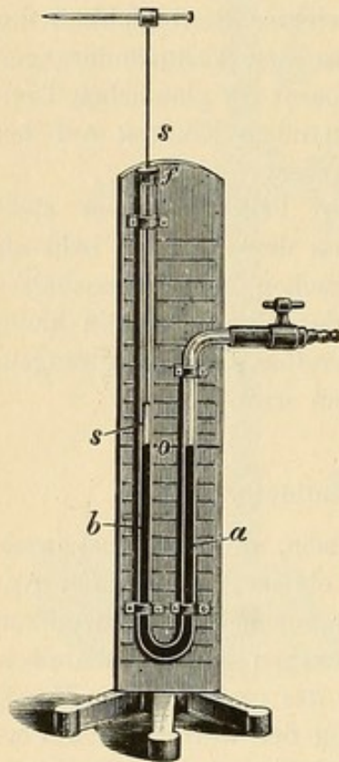
Fig. 52. Registrirendes Quecksilbermanometer. ( \frac{1}{3} nat. Gr.)
