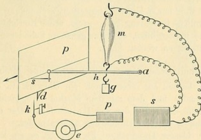
Fig. 224. Schema einer myographischen Vorrichtung.
