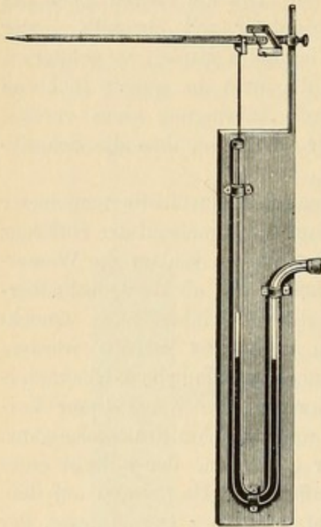
Fig. 53. Registrirendes Manometer mit Hebel- vergrösserung.
