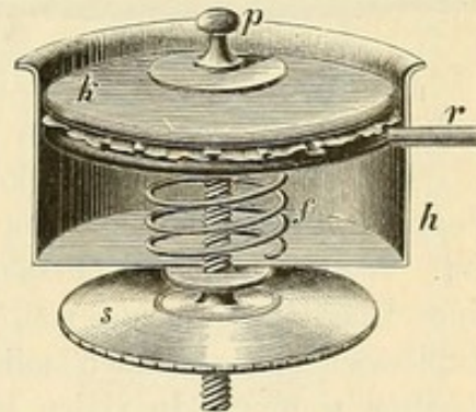
Fig. 155. Aufnahmekapsel des Marey'schen Kardiographen. ( \frac{1}{2} nat. Gr.)
