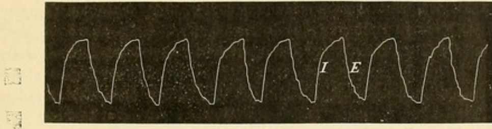
Fig. 222. Kaninchen. Vagi durchschnitten. Transmissions-Phrenograph.
