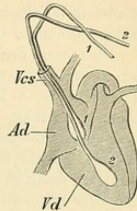
Fig. 153. Lage der kardiographischen Sonden im Herzen.
