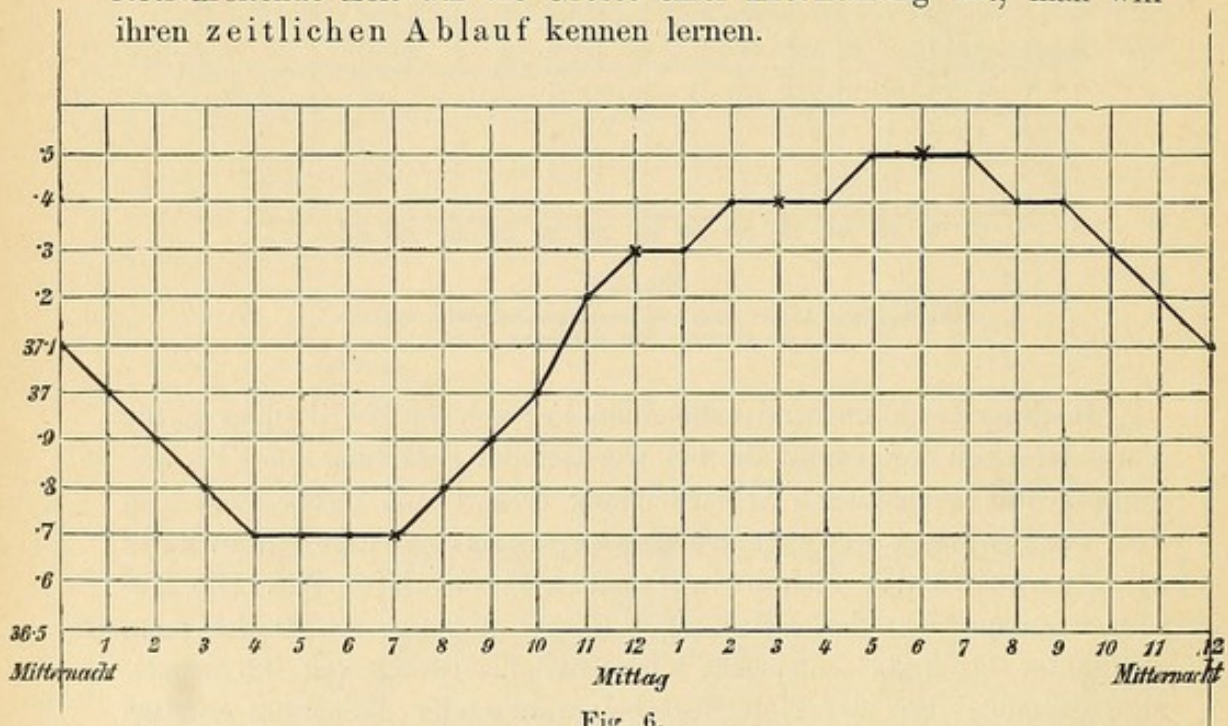
Fig. 6. Tägliche Temperaturschwankungen des Menschen. (Die mit * bezeichneten Stellen entsprechen den Mahlzeiten.)
