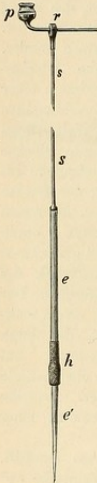
Fig. 163. Manometer-Schwimmer ( \frac{1}{2} nat. Gr.)
