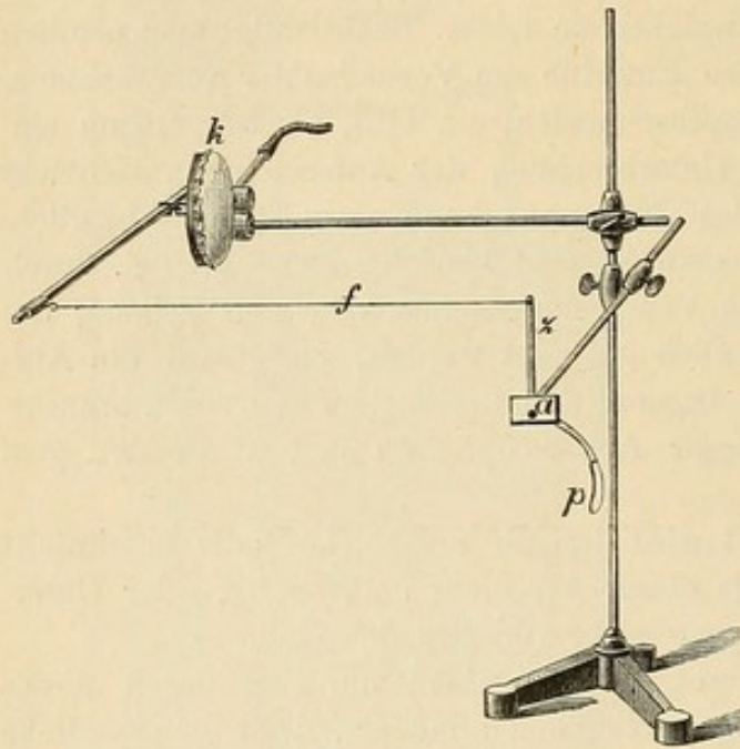
Fig. 221. Transmissions-Phrenograph ( \frac{1}{3} nat. Gr.)
