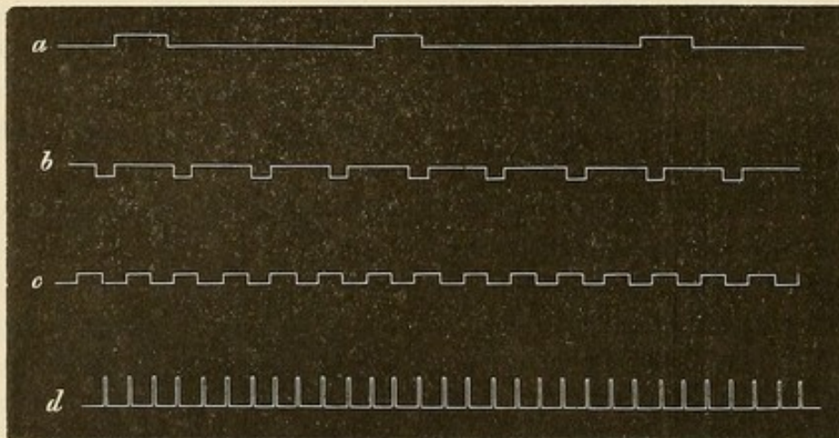
Fig. 100. Chronogramme (Fünfskundenmarken).
