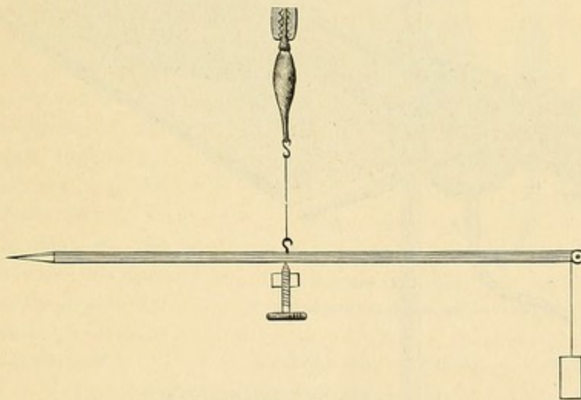
Fig. 242. Ueberlastungsverfahren.
