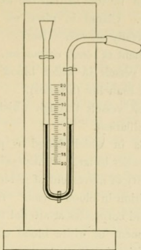
FIG. 152.—Manometer.
