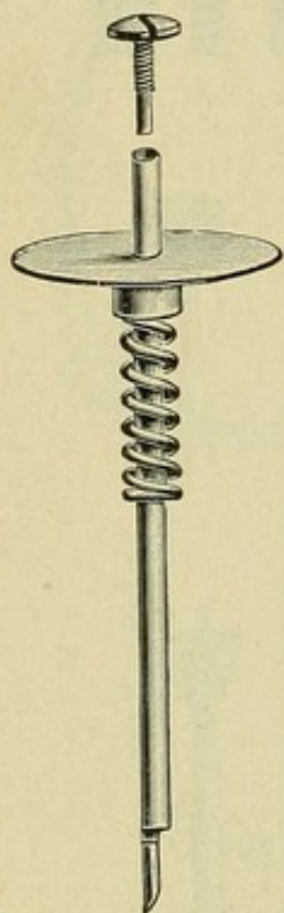
FIG. 84.—Disk mandrel.
