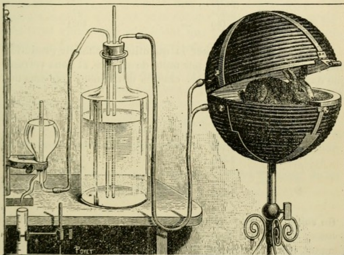
Fig. 30. — Calorimètre à siphon.
