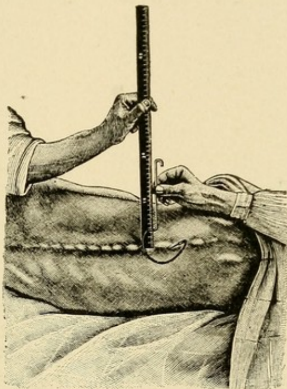
FIG. 39. (After Quinke.)
