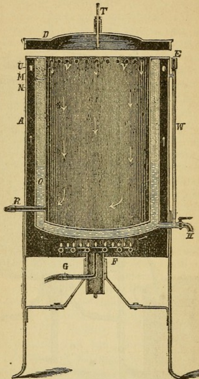
Dampfsterilisator für Verbandstoffe. Durchschnitt.
