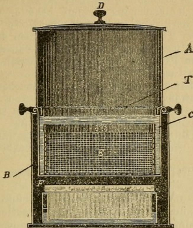
Combinirter Sterilisationsapparat für Instrumente und Verbandstoffe nach Schimmelbusch. Durchschnitt.
