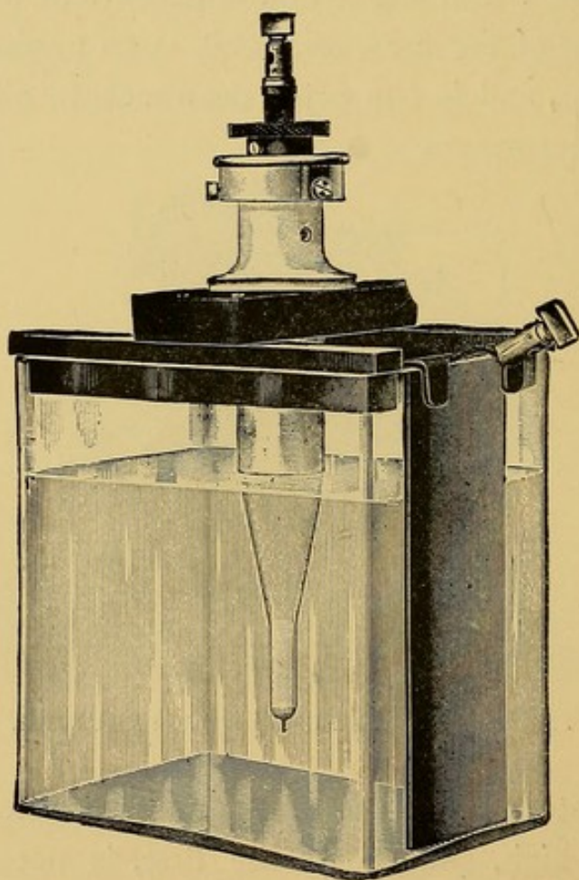
FIG. 17.—WEHNELT INTERRUPTER.
