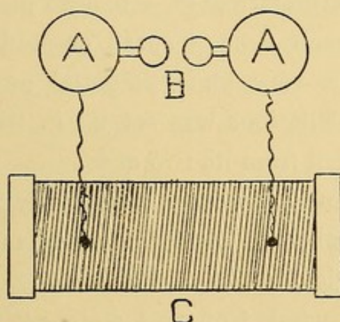
FIG. 1.—HERTZ' OSCILLATOR.
