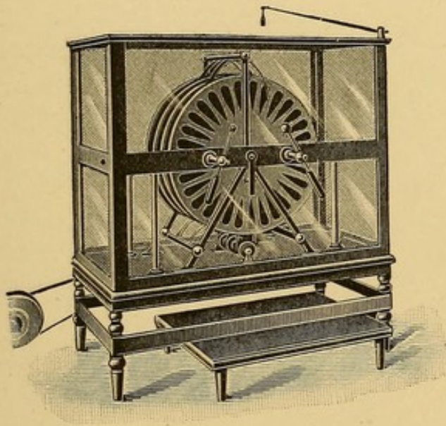
FIG. 26.—GLASS-PLATE STATIC MACHINE.
