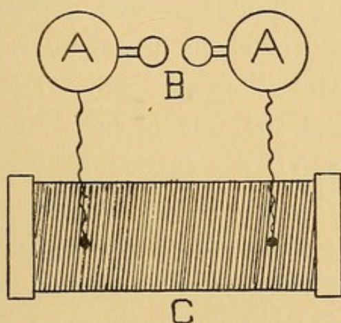
FIG. 29.—HERTZ' OSCILLATOR.
