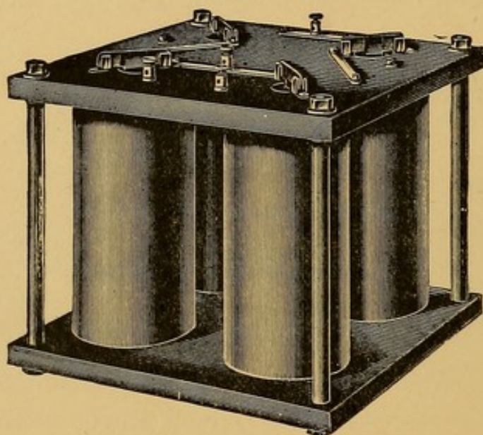
FIG. 23.—NODON VALVE.
