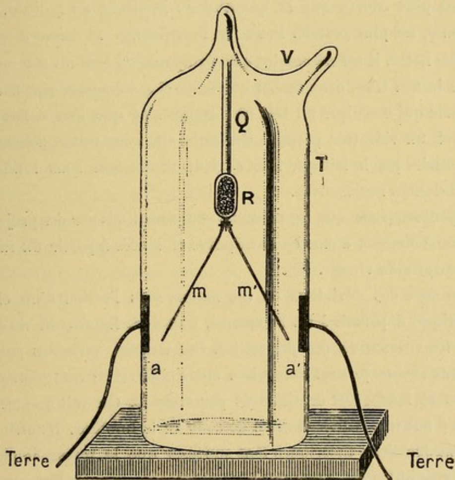
FIG. 22. — Appareil de Strutt à mouvement perpétuel.
