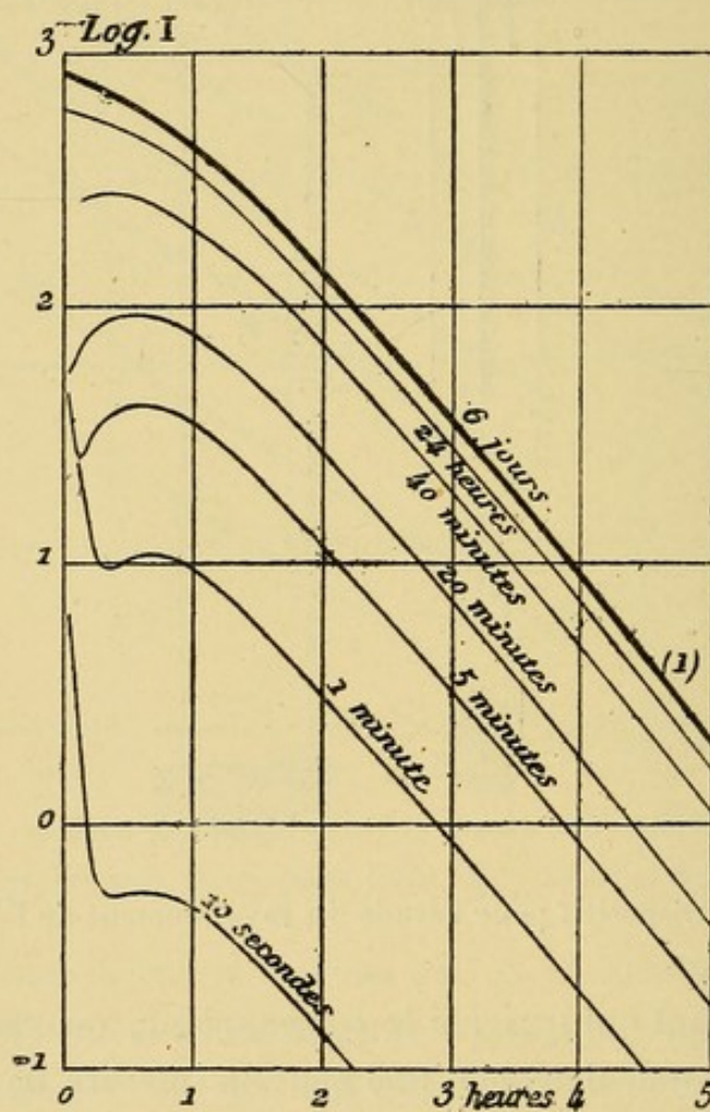
FIG. 31. — Influence de la durée d'activation sur la loi de désactivation.
