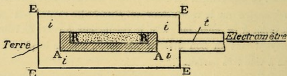
FIG. 21. — Appareil pour l'étude des rayons \beta .
