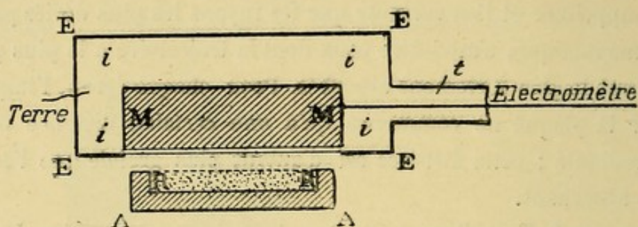
FIG. 20. — Appareil pour l'étude des rayons \beta .
