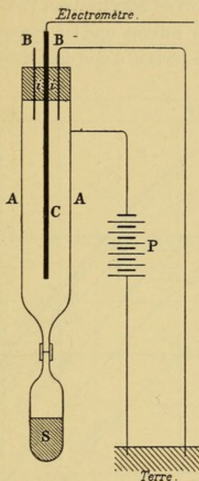
FIG. 30. — Dispositif pour l'étude du rayonnement de l'émanation.
