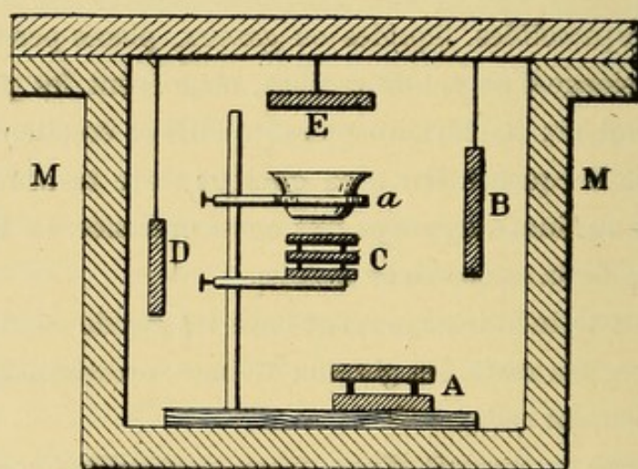
FIG. 26. — Activation des corps dans une enceinte fermée.
