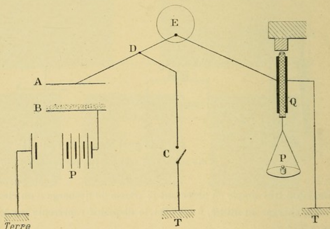
FIG. 9. — Dispositif employé dans la méthode électrométrique.
