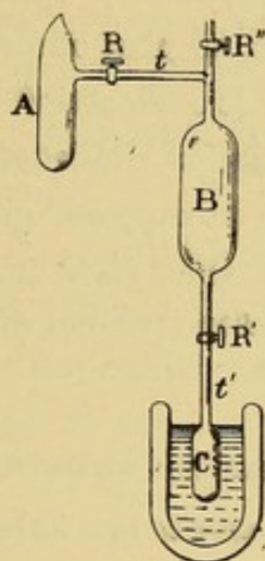
FIG. 35. — Condensation de l'émanation dans l'air liquide.
