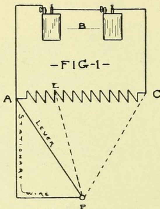
Fig. 13.—Diagram of rheostat. (Victor.)
