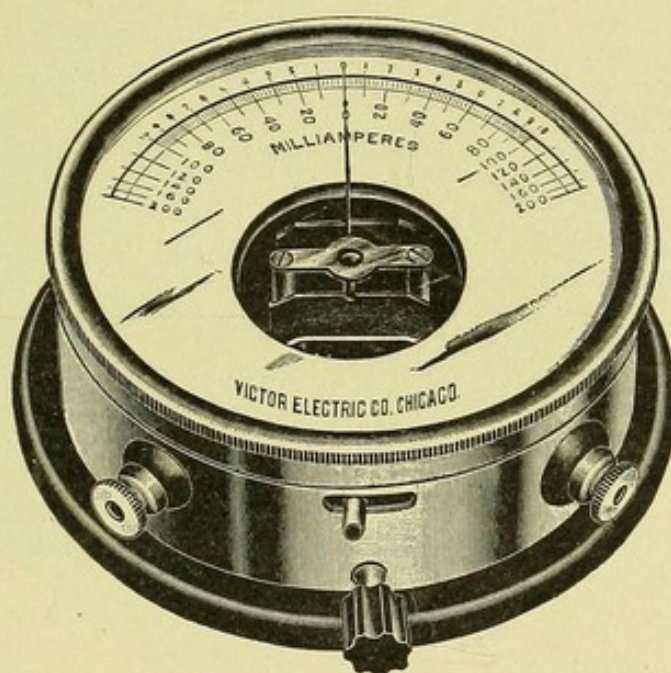
Fig. 10.—Milliampèremeter. (Victor.)
