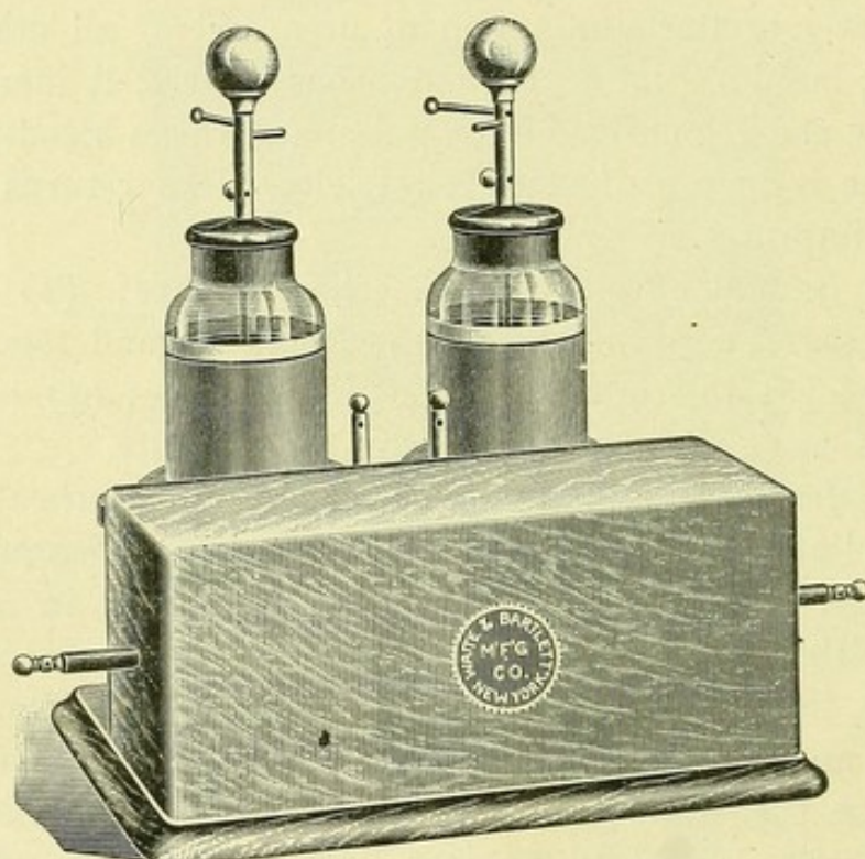
Fig. 39.—Leyden jar. (Waite and Bartlett.)
