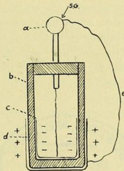
Fig. 40.—A Leyden jar.
