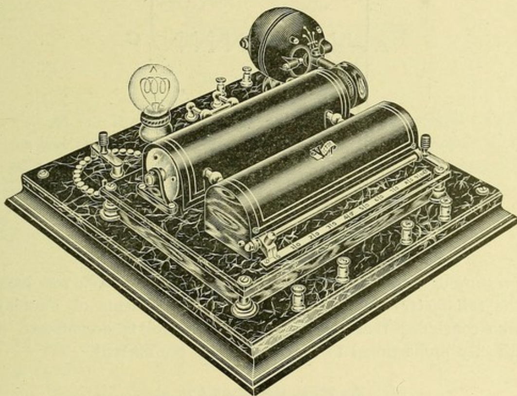
Fig. 12.—Multiplex. (Victor.)
