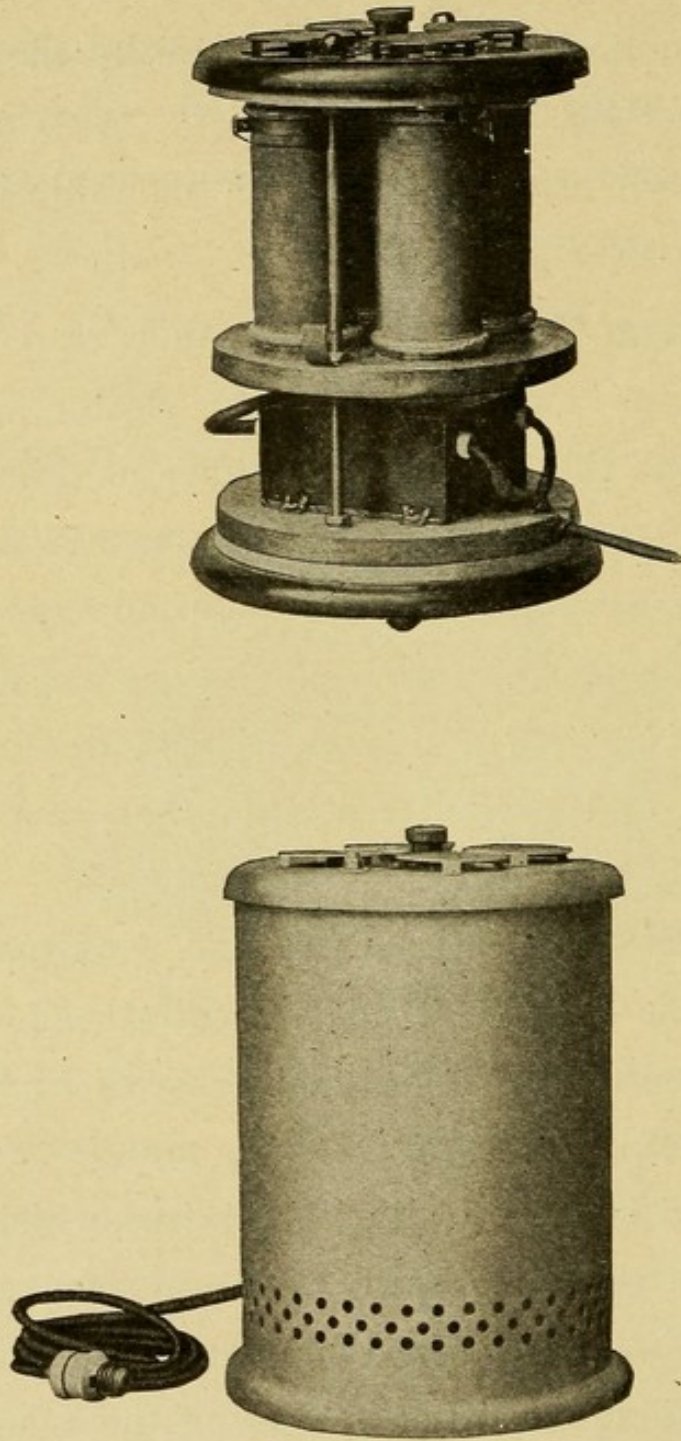
Fig. 59—Room Ozonizer.
