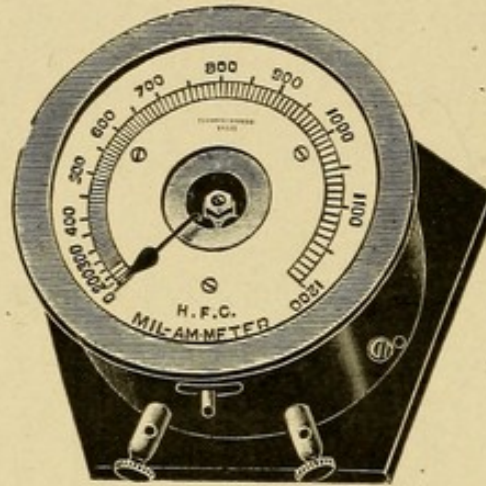
Fig. 16—Hot Wire Meter.
