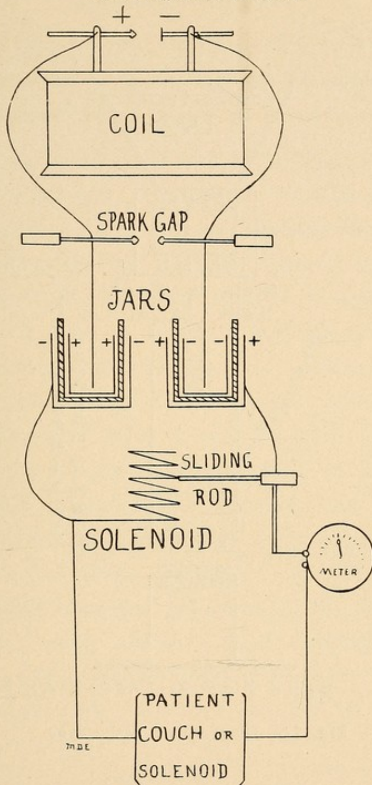
Fig. 13—Diagram of D'Arsonval Type.
