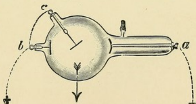
FIG. 2. — Ampoule de Crookes.
