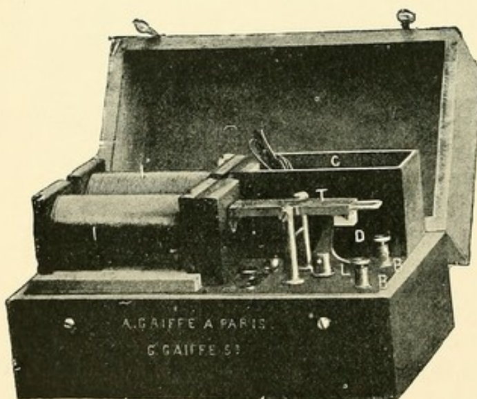
FIG. 20. — Appareil faradique portatif à hélices mobiles, du Dr A. Tripier.
