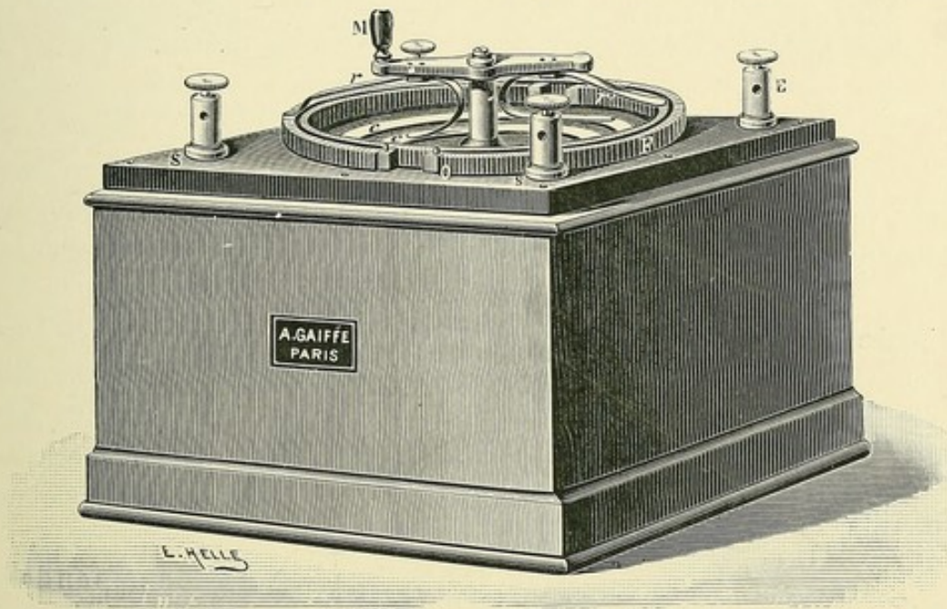
FIG. 18. — Réducteur de potentiel.
