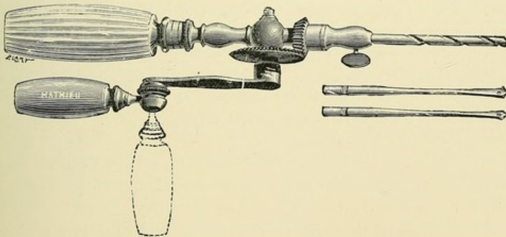
FIG. 22. — Perforateur à manivelle.
