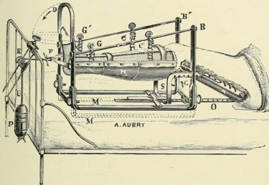
FIG. 62. — H, hamac jambier. — A, hamac crural. — G, fourche à crémaillère supportant le hamac crural. — GG' galets mobiles. — CC', chaînettes en échelle. — BB', cadre rectangulaire à base mobile pour rectifier le plan du matelas. — D, cerceau articulé avec le cadre. — E, poulie à coulisseaux mobiles sur les tiges en U. — P, poids cylindro-sphérique composé de disques-fenêtres de 1/2 et 1 kilogramme. — F, étrier auquel est fixée la corde qui supporte le poids. — MM, bandelettes mobiles dans le sens vertical pour rectifier le plan du matelas. — O, bandelette articulée à la base du cadre du hamac crural et percée de trous dans lesquels s'engage un crochet rivé à la branche horizontale de la base du cadre rectangulaire.
