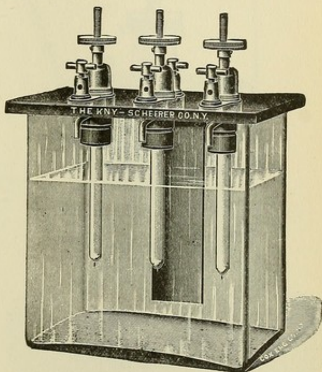
FIG. 74.—Wehnelt interrupter.
