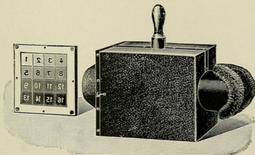
FIG. 219.—The skiameter.
