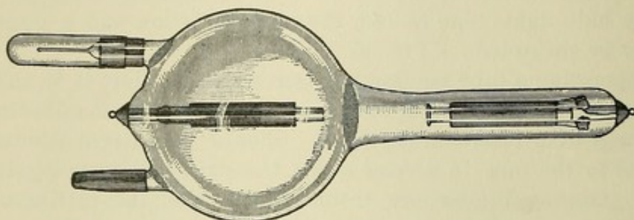
FIG. 95.—Villard's ventril tube.
