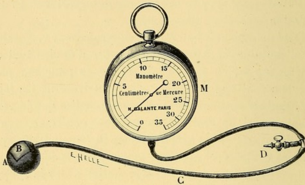
Fig. 1. — Sphygmomanomètre.
