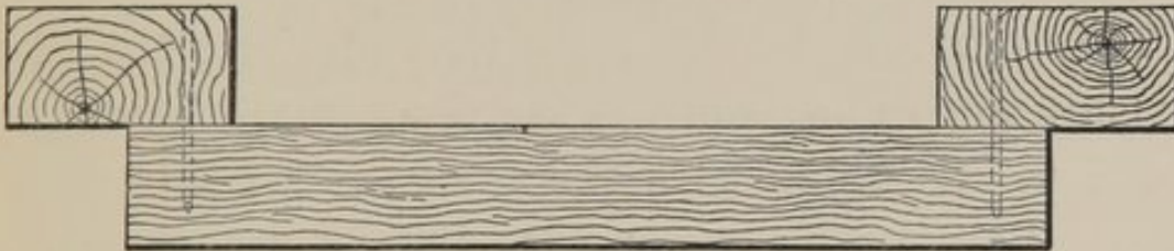
Fig. 1—PLANK BOTTOM
