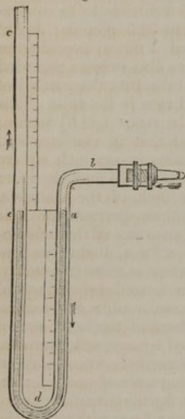
Hæmadynamometer.
