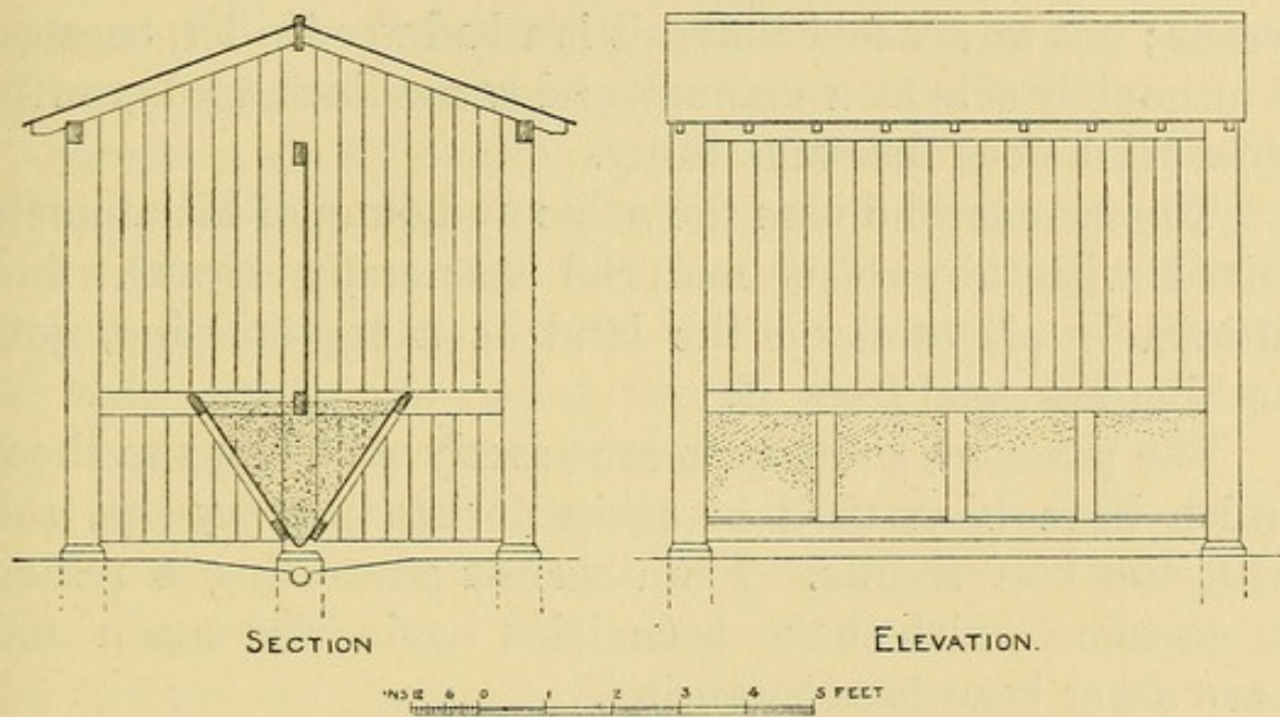
FIG. 21.—DRY URINAL.
