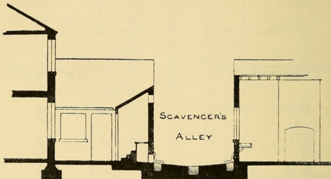
FIG. 30.—SECTION A-A.
