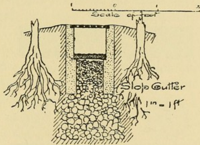
FIG. 26.—FILTRATION GUTTER.
