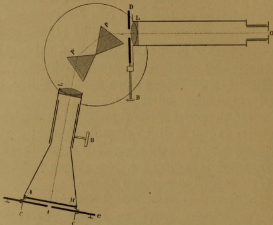
Fig. 1. — Spectroscope modifié.
