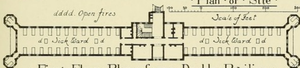
· First · Floor · Plan · of · one · Double · Pavilion ·
