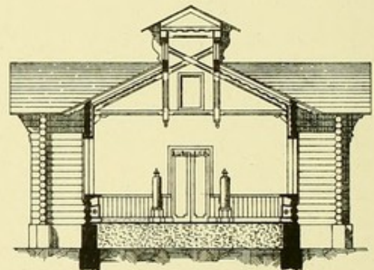
· Section on Line A·B ·
