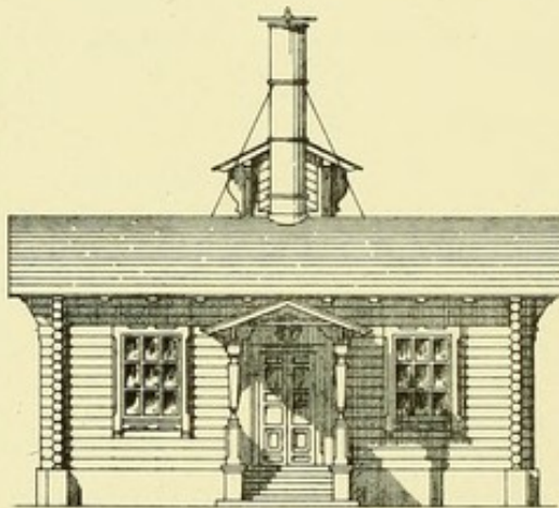
· End · Elevation ·
