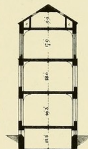
:Section:on:line:AB:
