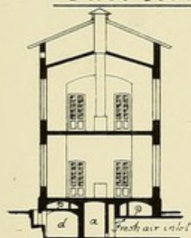
· Section on Line AB ·
