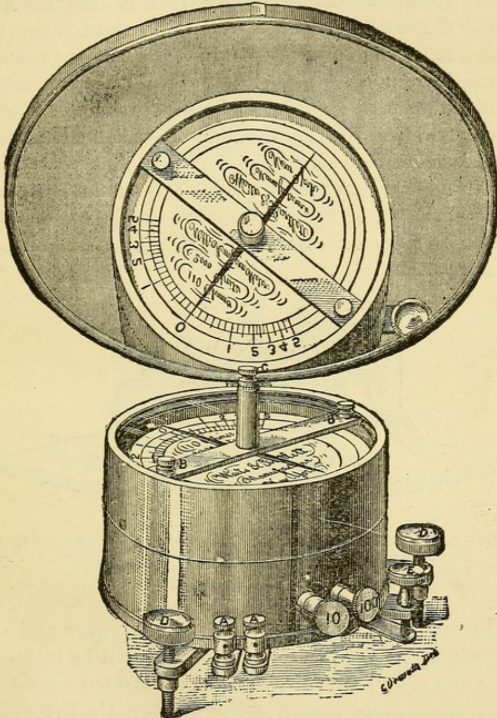
FIG. 6.—WAITE & BARTLETT'S MILLIAMPÈRE METER.
