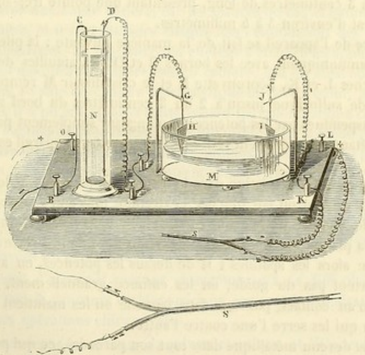
FIG. 25. — Appareil collecteur de A. Thenard.
