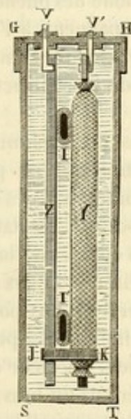
Fig. 49. — Couple au chlorure d'argent de Gaiffe (**).
