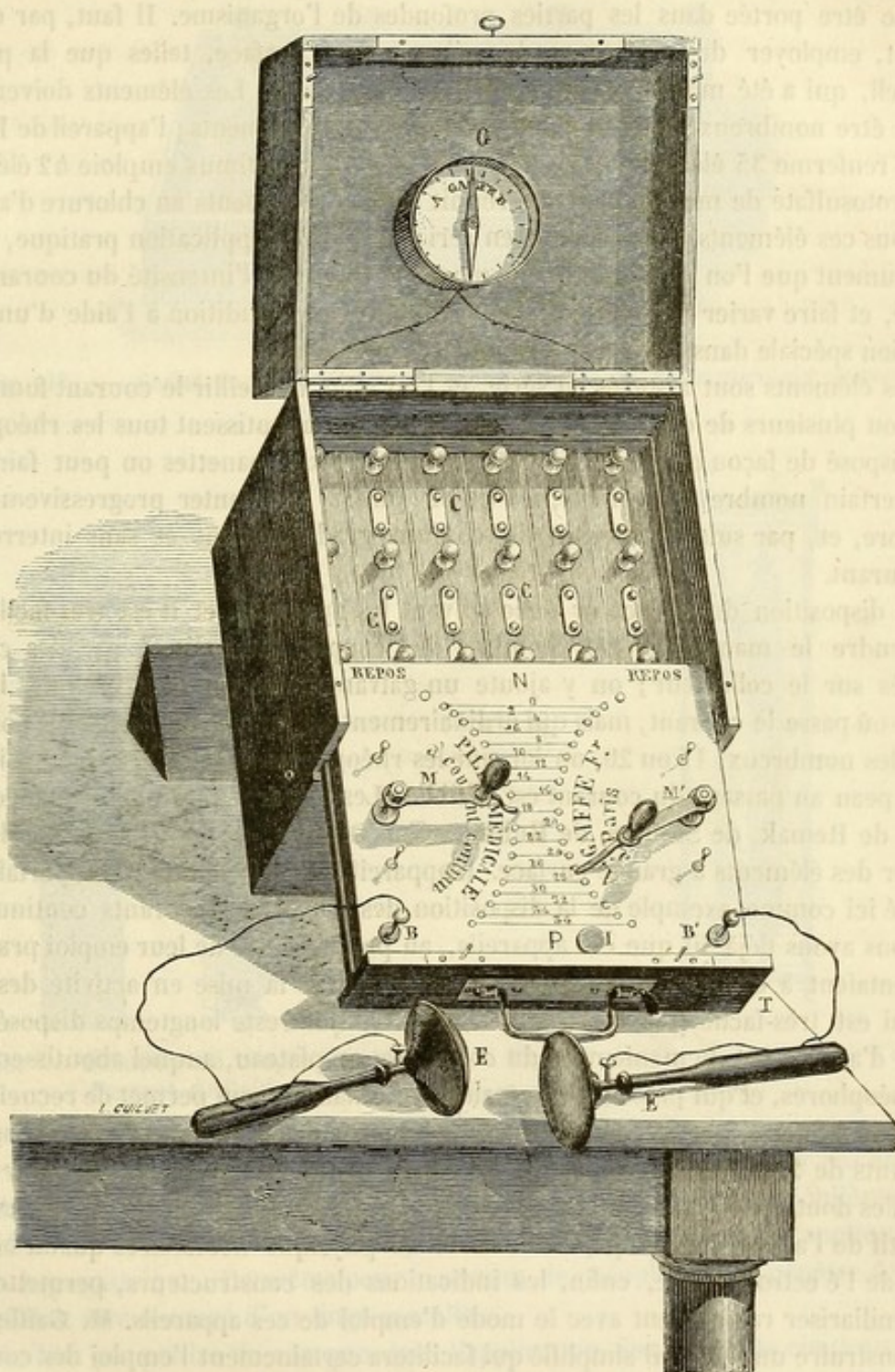
Fig. 46. — Pile portative à courant continu de Gaiffe (*).
