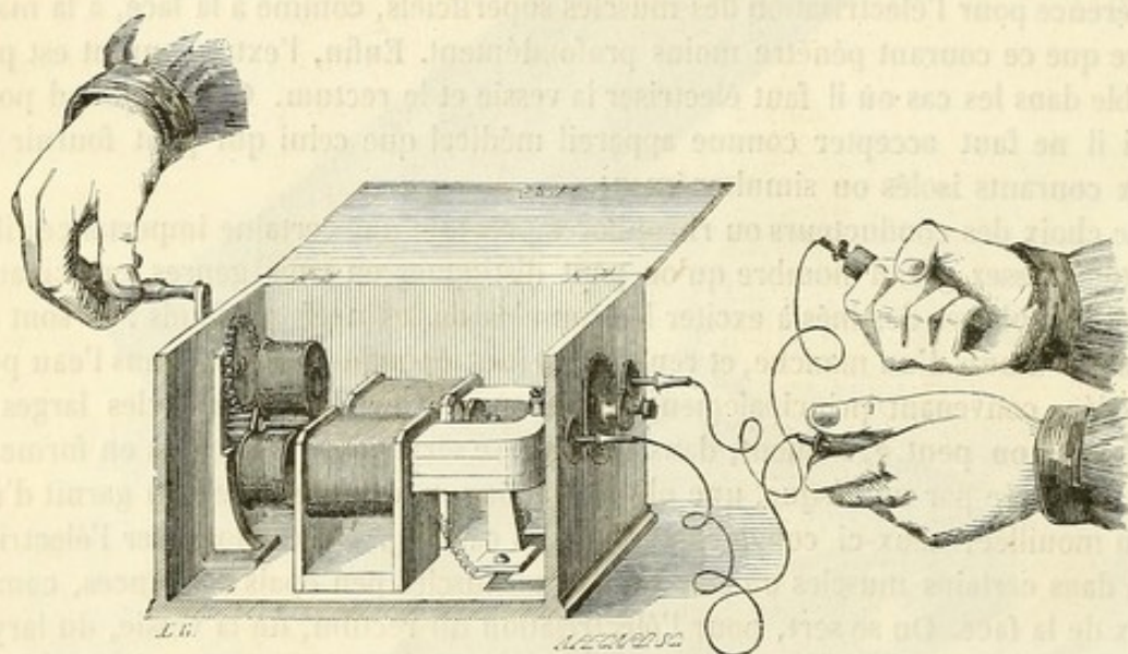
Fig. 45. — Appareil magnéto-électrique de Gaiffe.
