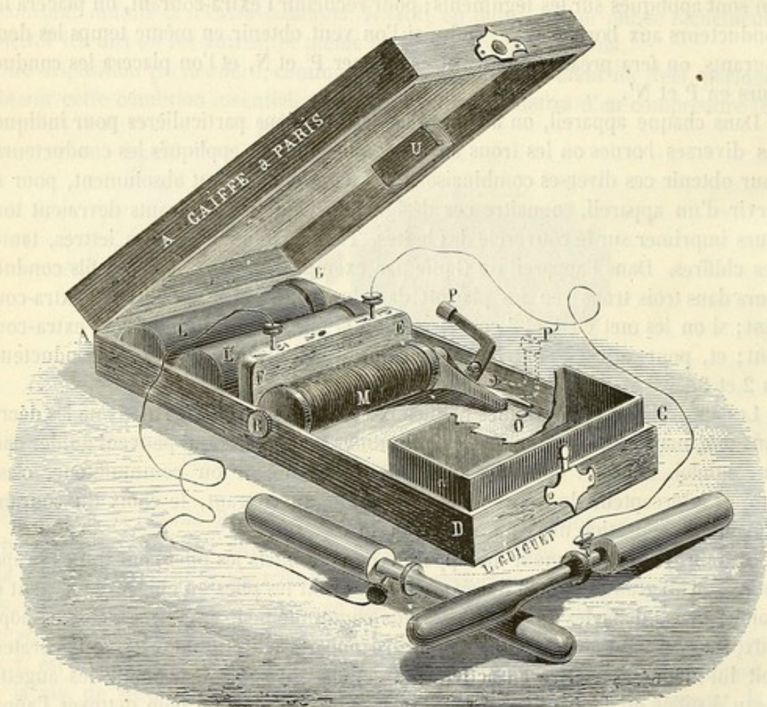
Fig. 45. — Appareil volta-faradique de Gaiffe (*).
