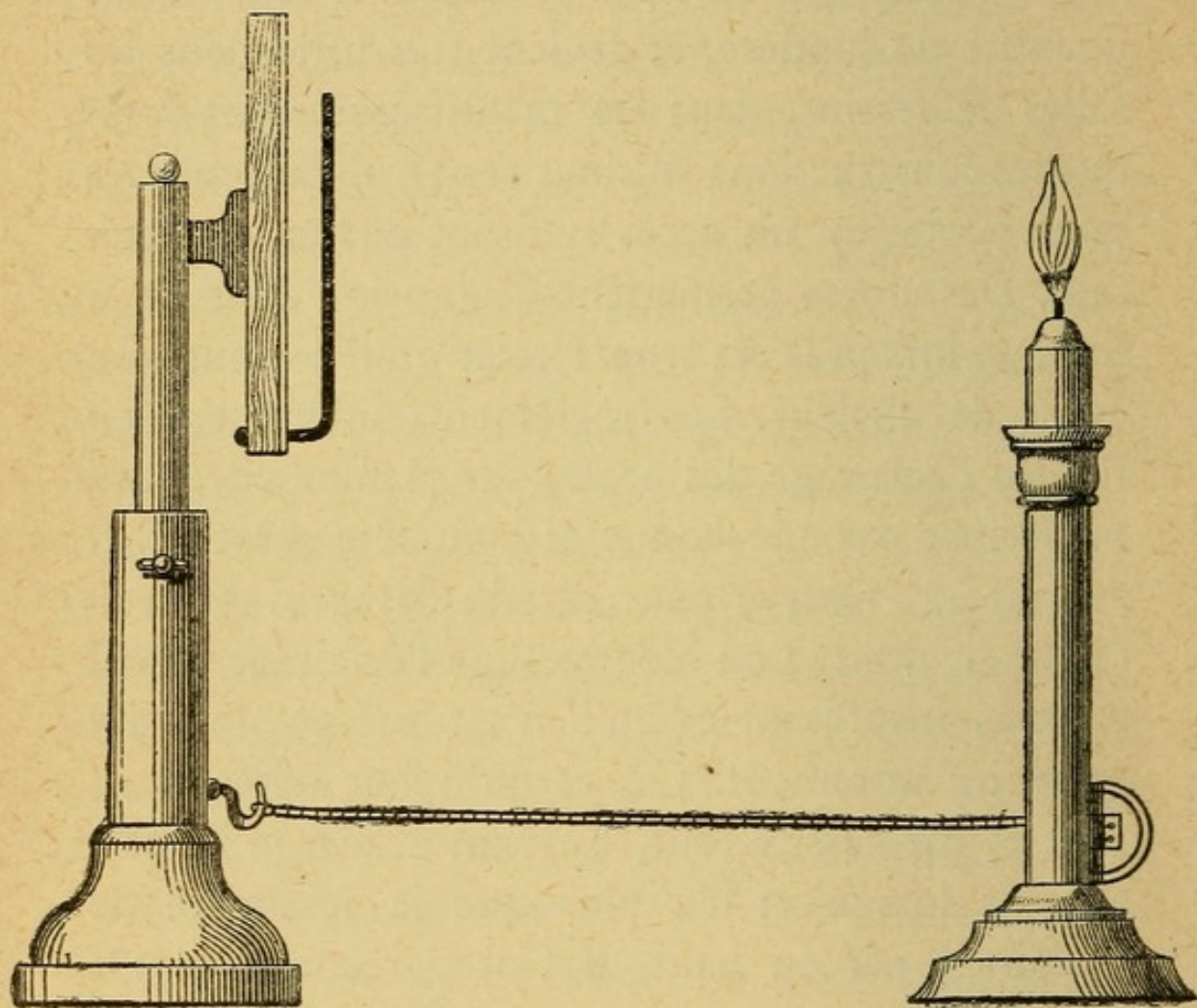
Fig. 32. — Photomètre de Bertin-Sans.
