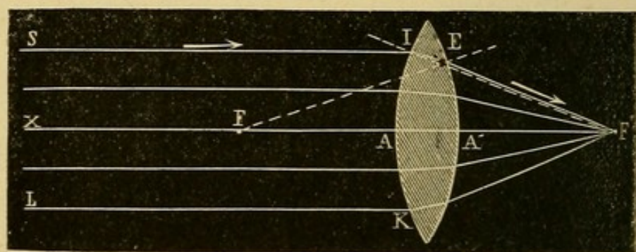
Fig. 16. — Foyer principal d'une lentille biconvexe*.
