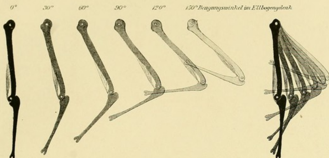
Beugebewegung des Arms ohne Handbelastung infolge alleiniger Wirkung eines eingelenkigen Beugemuskels des Ellbogengelenks.
