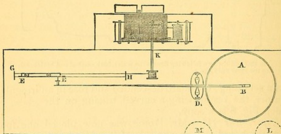
FIG. 9. (Plan.)
